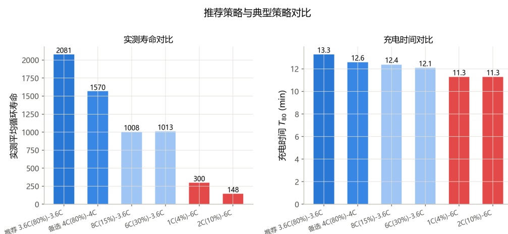
图 18 推荐策略与典型策略的实测寿命与充电时间对比
