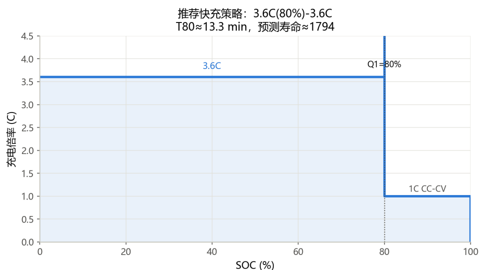
图 17 推荐快充策略电流剖面 (3.6C(80%)-3.6C)
