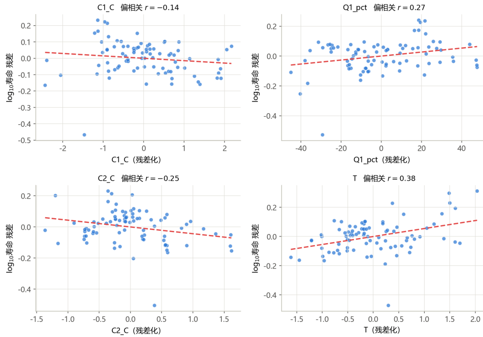
偏回归图（控制其他变量与批次后，各参数与寿命的关系）
