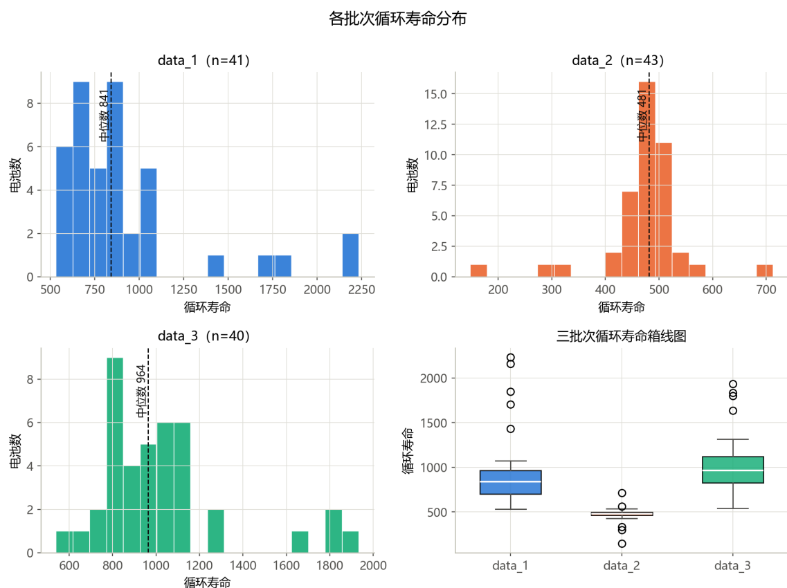
图2 各批次循环寿命分布直方图
