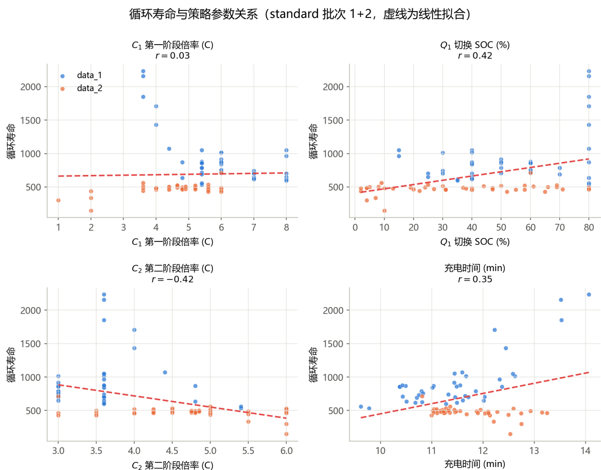
图 4 cycle_life 与各策略参数关系 (standard 批次)
