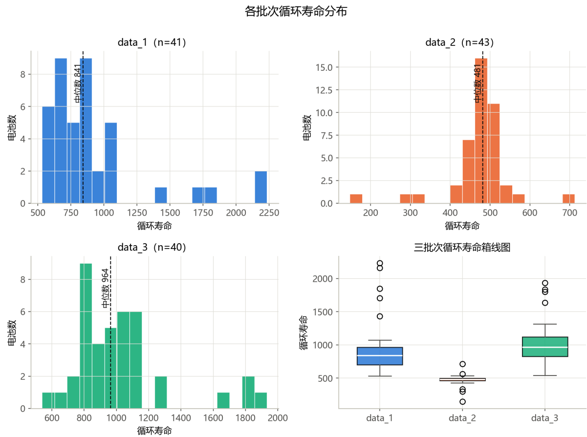
图 2 各批次循环寿命分布直方图
