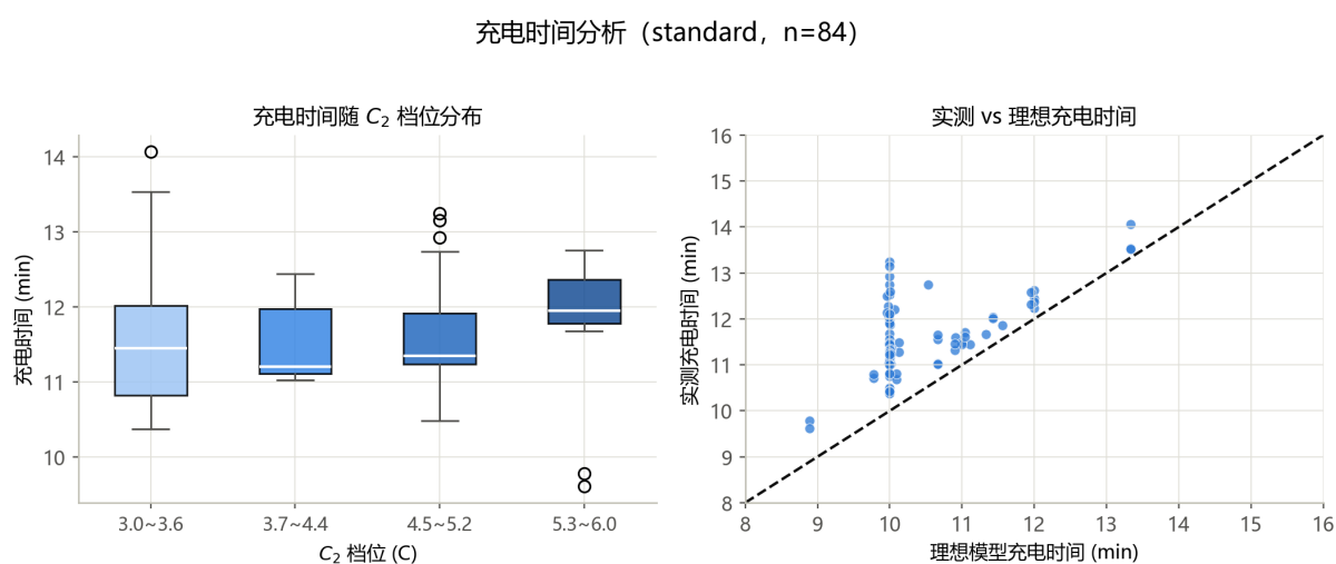
图 6 充电时间分析：随 C_2 档位分布与理想模型对比 (standard, n=84)
