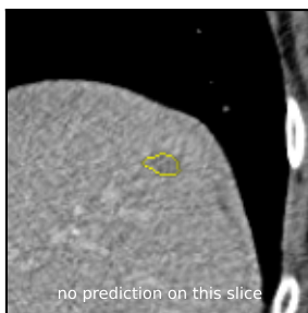
ResEnc-M DSC 0.000
