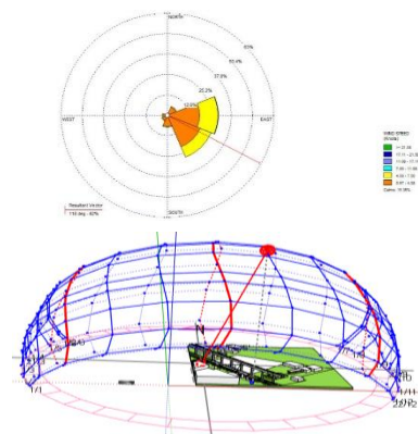
Gambar 4. Analisa Matahari pada site
