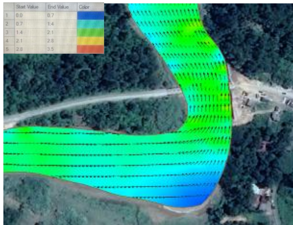
Gambar 4. Pola arah arus pada jembatan air enim 3 kondisi Eksisting
