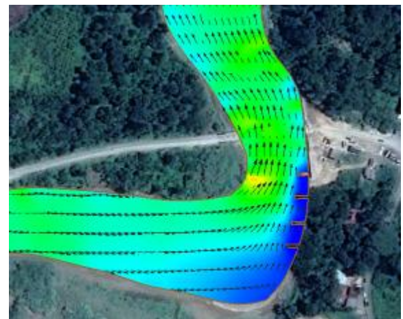
Gambar 6. Pola kecepatan arus pada jembatan air enim 3 kondisi ada krib
