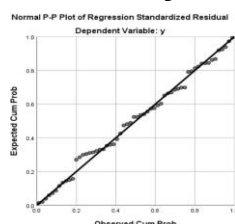
Gambar 4.9 Hasil Uji Normalitas
