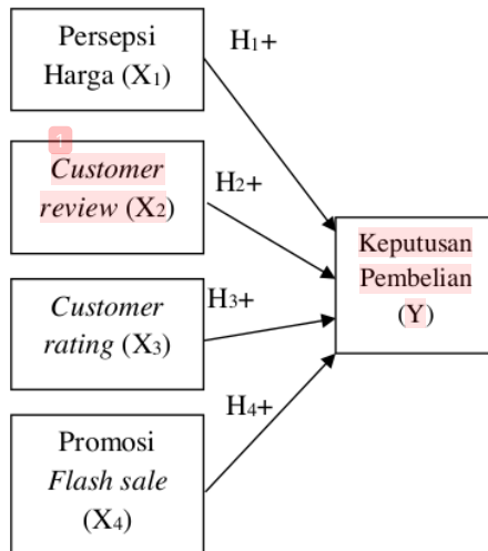
Gambar 1 Kerangka Pemikiran
