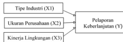
Gambar 1 Kerangka Teoritis
