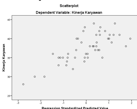
Gambar 4.3 Uji Heteroskedasitas
