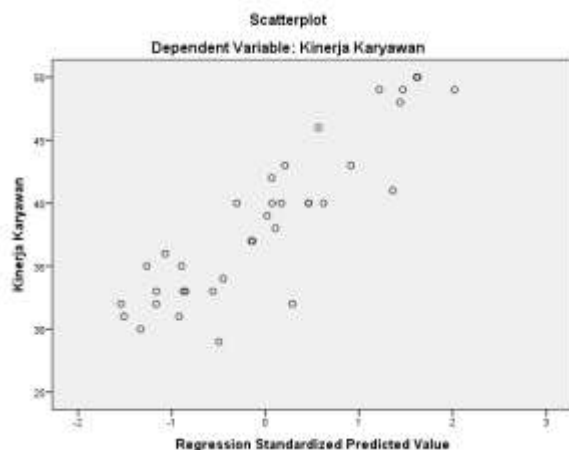
Gambar 1 Uji Heteroskedasitas
