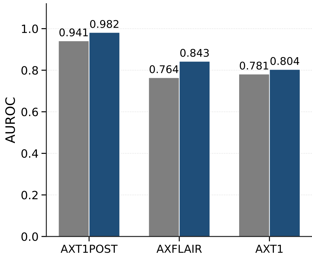
Volume-level AUROC
