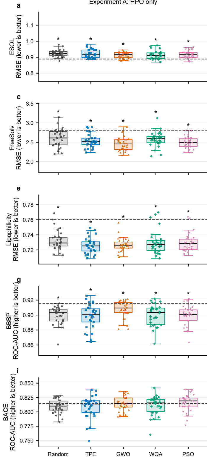
Experiment A: HPO only
