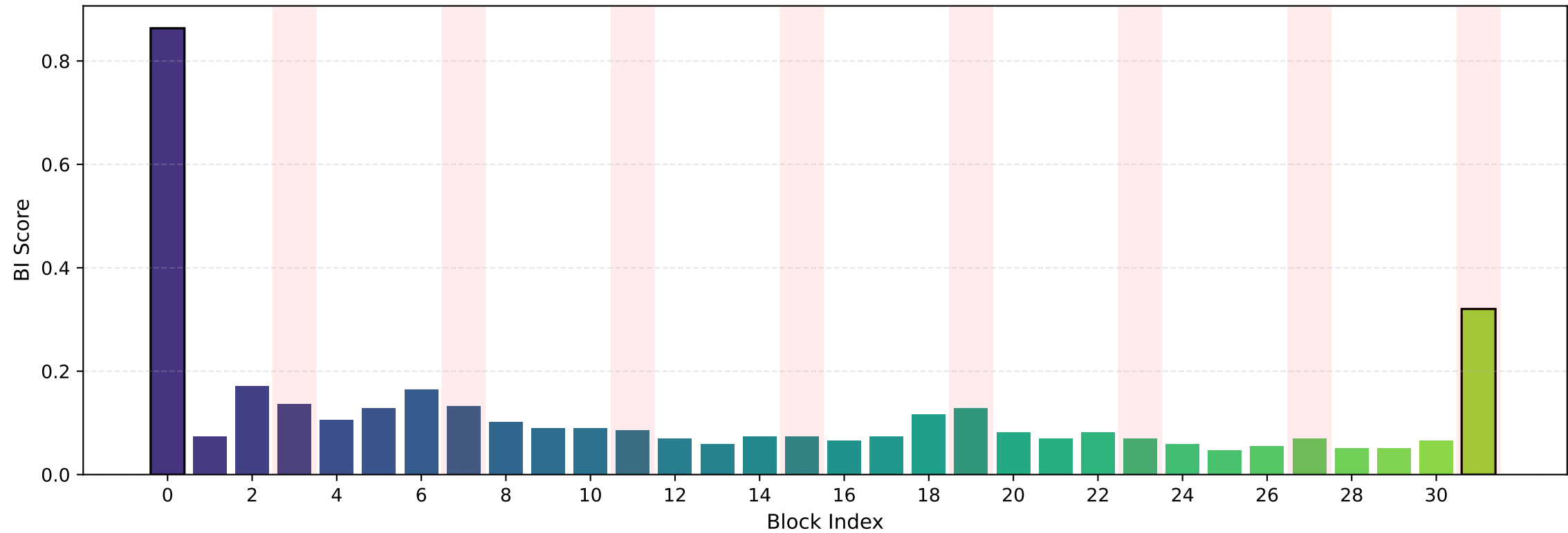
Qwen3.5-4B BI per Block
