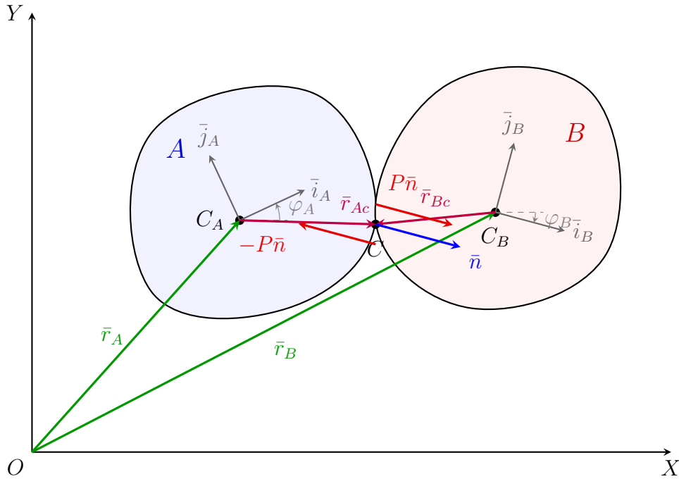
Figura 7: Reprezentarea coliziunii între două corpuri rigide A și B . Punctul de contact C este definit prin vectorii de poziție relativi \vec{r}_{Ac} și \vec{r}_{Bc} . Interacțiunea generează percuțiile +P\vec{n} și -P\vec{n} care acționează de-a lungul normalei de coliziune \vec{n} .
