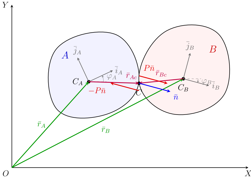
Figure 7: Reprezentarea coliziunii între două corpuri rigide A și B. Punctul de contact C este definit prin vectorii de poziție relativi \vec{r}_{Ac} și \vec{r}_{Bc} . Interacțiunea generează percuțiile +P\vec{n} și -P\vec{n} care acționează de-a lungul normalei de coliziune \vec{n} .
