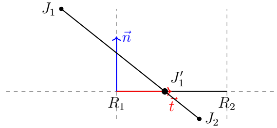
Figure 5: Reprezentarea tăierii laturii incidente în raport cu planul de referință.
