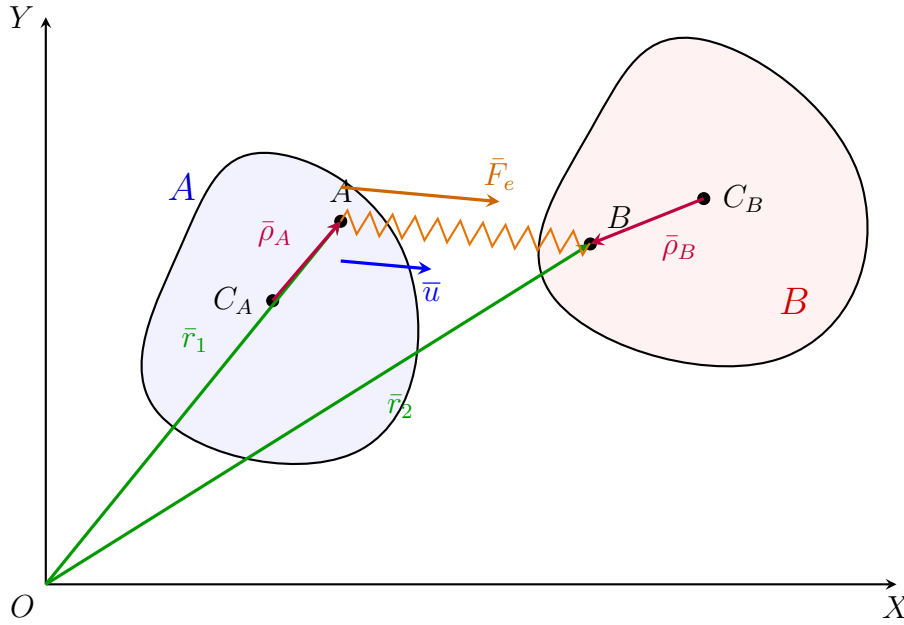
Figure 2: Reprezentarea unui arc elastic, interacționând între punctele de prindere A și B a două corpuri rigide distincte.
