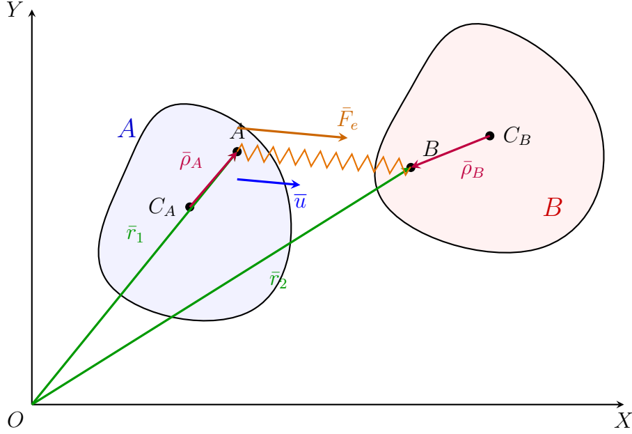
Figura 2: Reprezentarea unui arc elastic, interacționând între punctele de prindere A și B a două corpuri rigide distincte.
