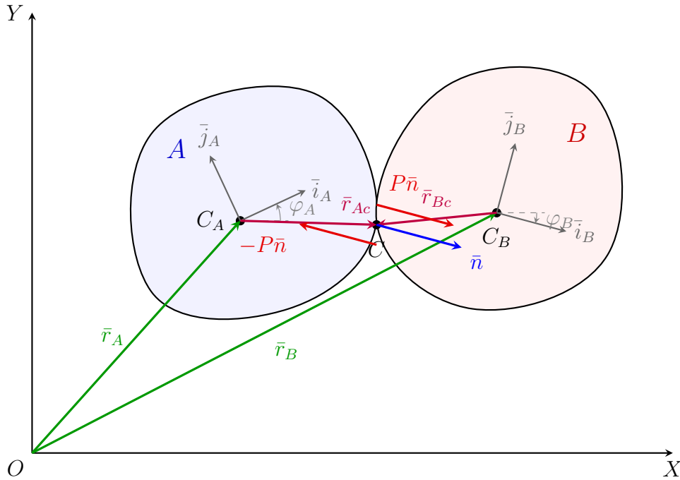
Figura 7: Reprezentarea coliziunii între două corpuri rigide A și B. Punctul de contact C este definit prin vectorii de poziție relativi \vec{r}_{Ac} și \vec{r}_{Bc} . Interacțiunea generează percuțiile +P\vec{n} și -P\vec{n} care acționează de-a lungul normalei de coliziune \vec{n} .
