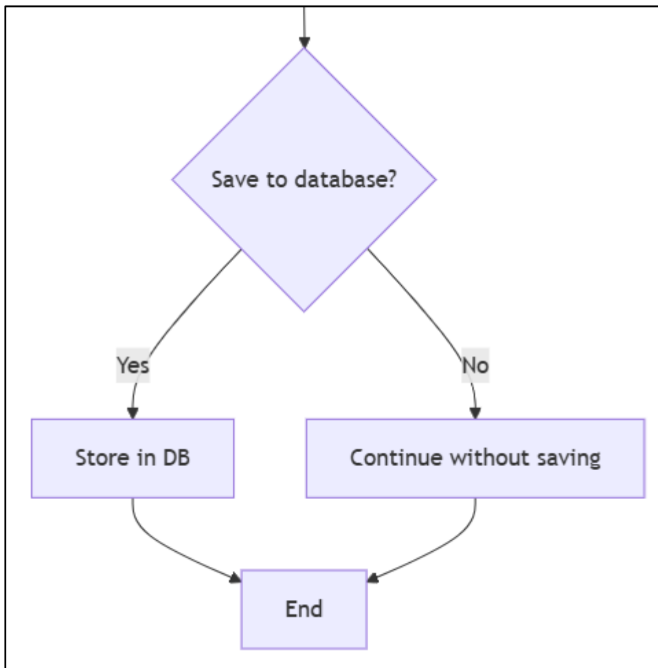
Abbildung 23 - Ablaufdiagramm Teil 3
