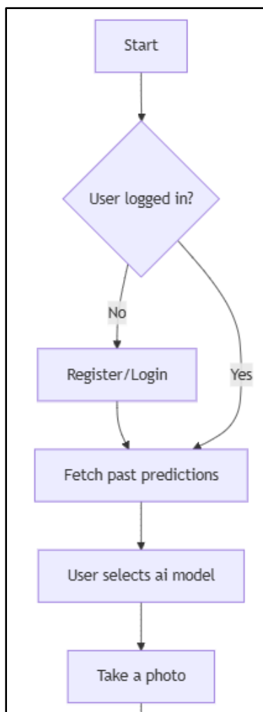
Abbildung 22 - Ablaufdiagramm Teil 1
