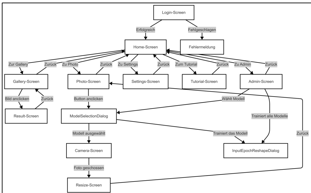
Abbildung 27: Flowchart
