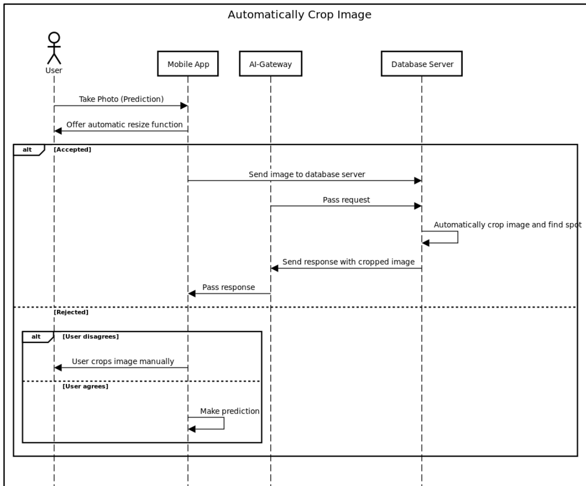
Abbildung 11 - Sequenzdiagramm: Automatisches Zuschneiden von Bildern
