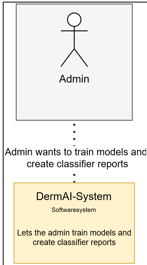
Abbildung 18 - C4-Context-Admin
