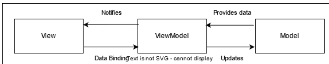
Abbildung 24 - MVVM-Architektur
