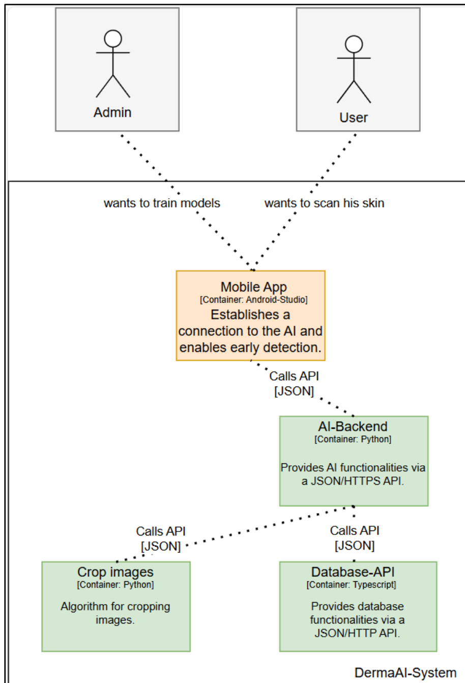
Abbildung 19 - C4-Container
