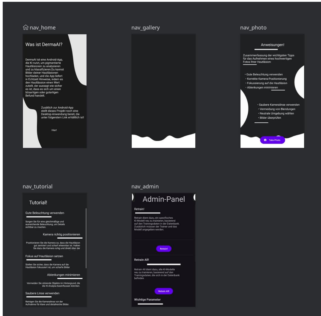
Abbildung 26: Navigation
