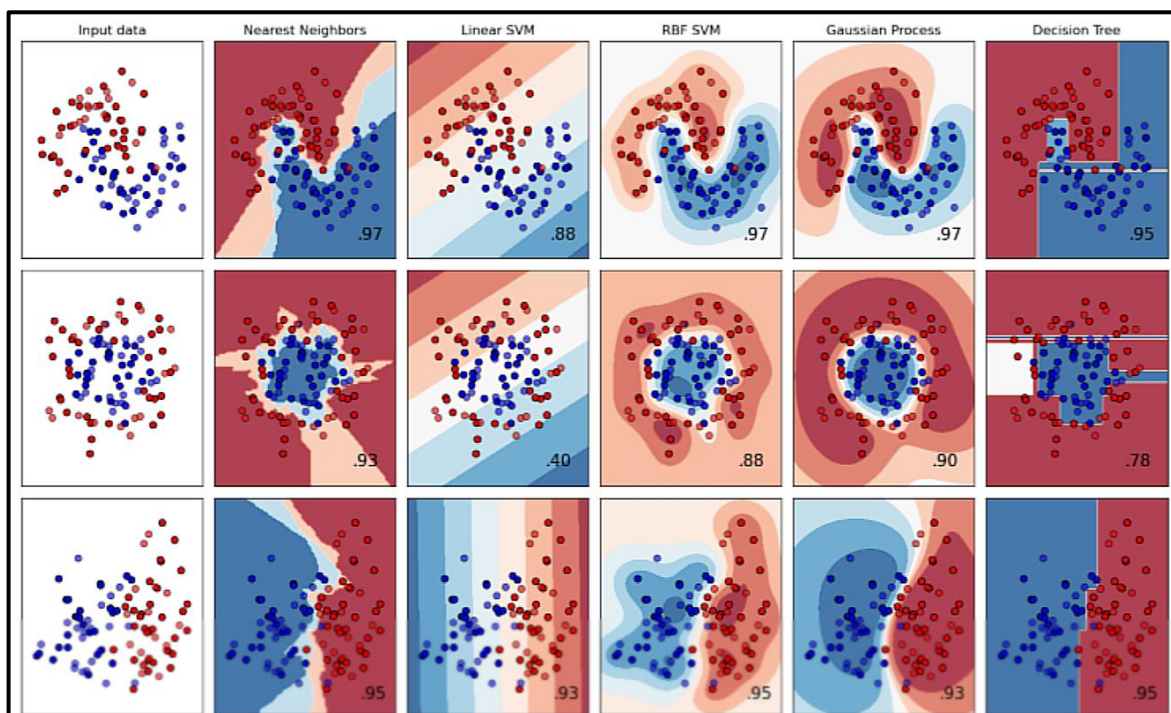
Abbildung 2 - Classifier Comparison
