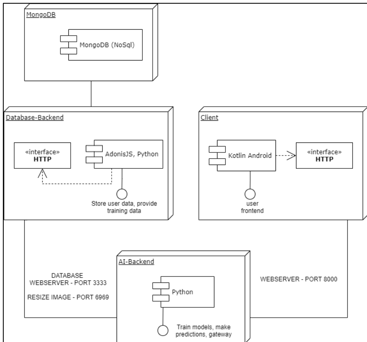
Abbildung 15 - Komponentendiagramm
