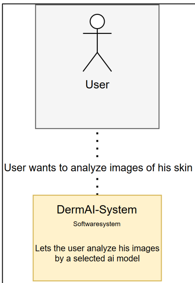
Abbildung 17 - C4-Context-User
