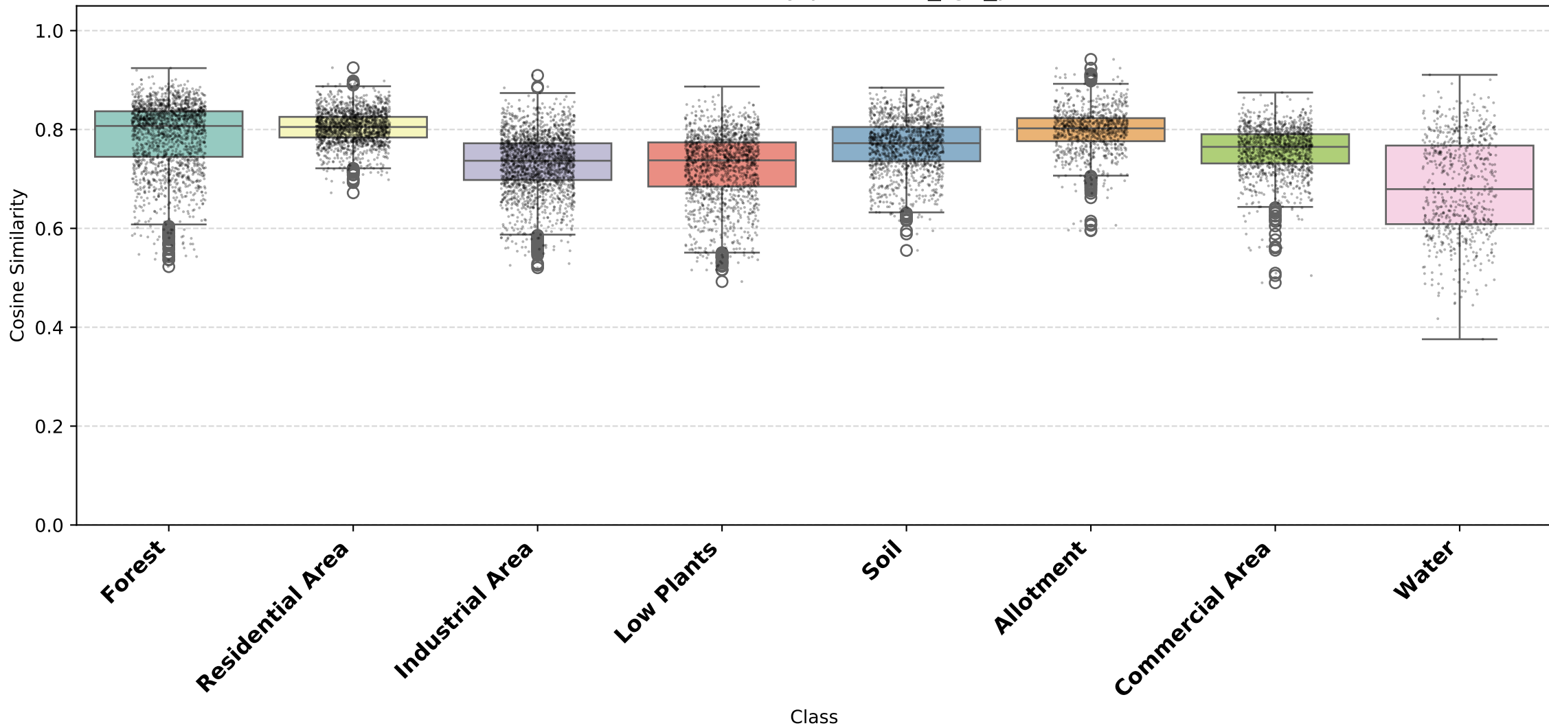
Cosine Similarity per Class_rgb_pca
