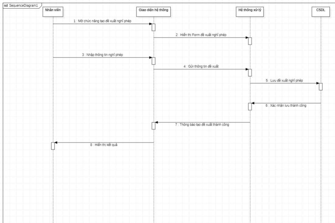
Hình 3.2. Sequence Diagram của chức năng tạo đề xuất nghỉ phép
