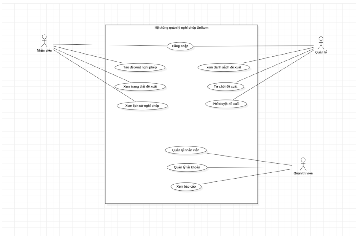
Hình 3.1. Use Case Diagram của hệ thống quản lý nghỉ phép Unikom
