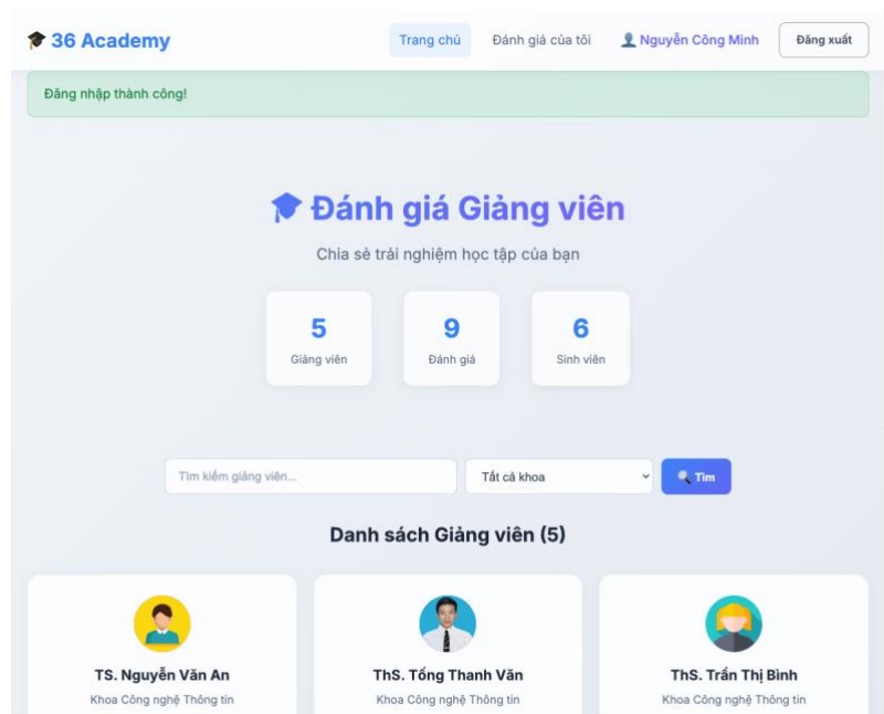
Hình 4-4: Giao diện trang chủ sau khi đăng nhập
