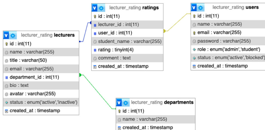
Hình 3-16: ERD của hệ thống đánh giá giảng viên
