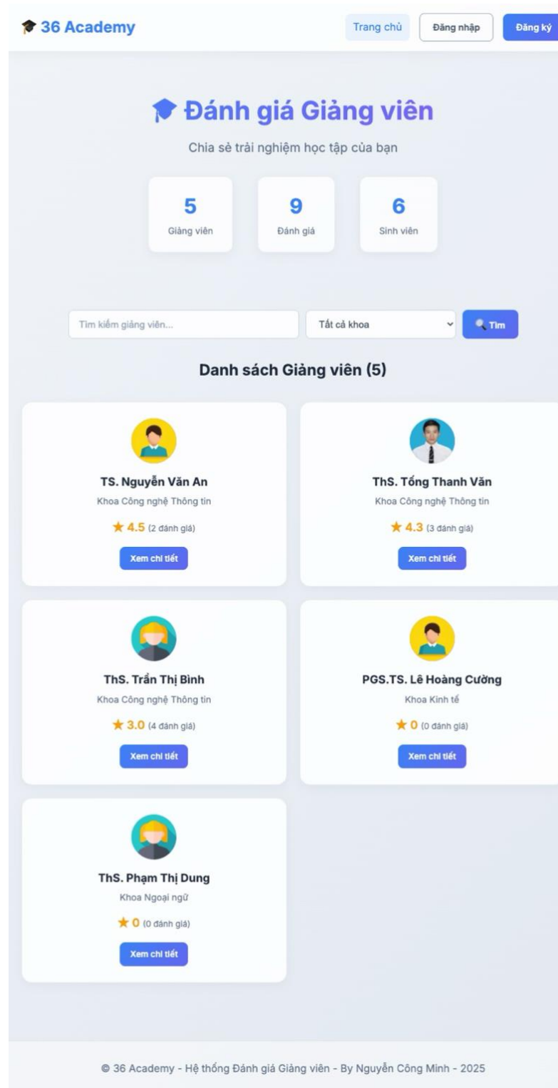
Hình 4-1: Giao diện trang chủ (Guest - Chưa đăng nhập)
