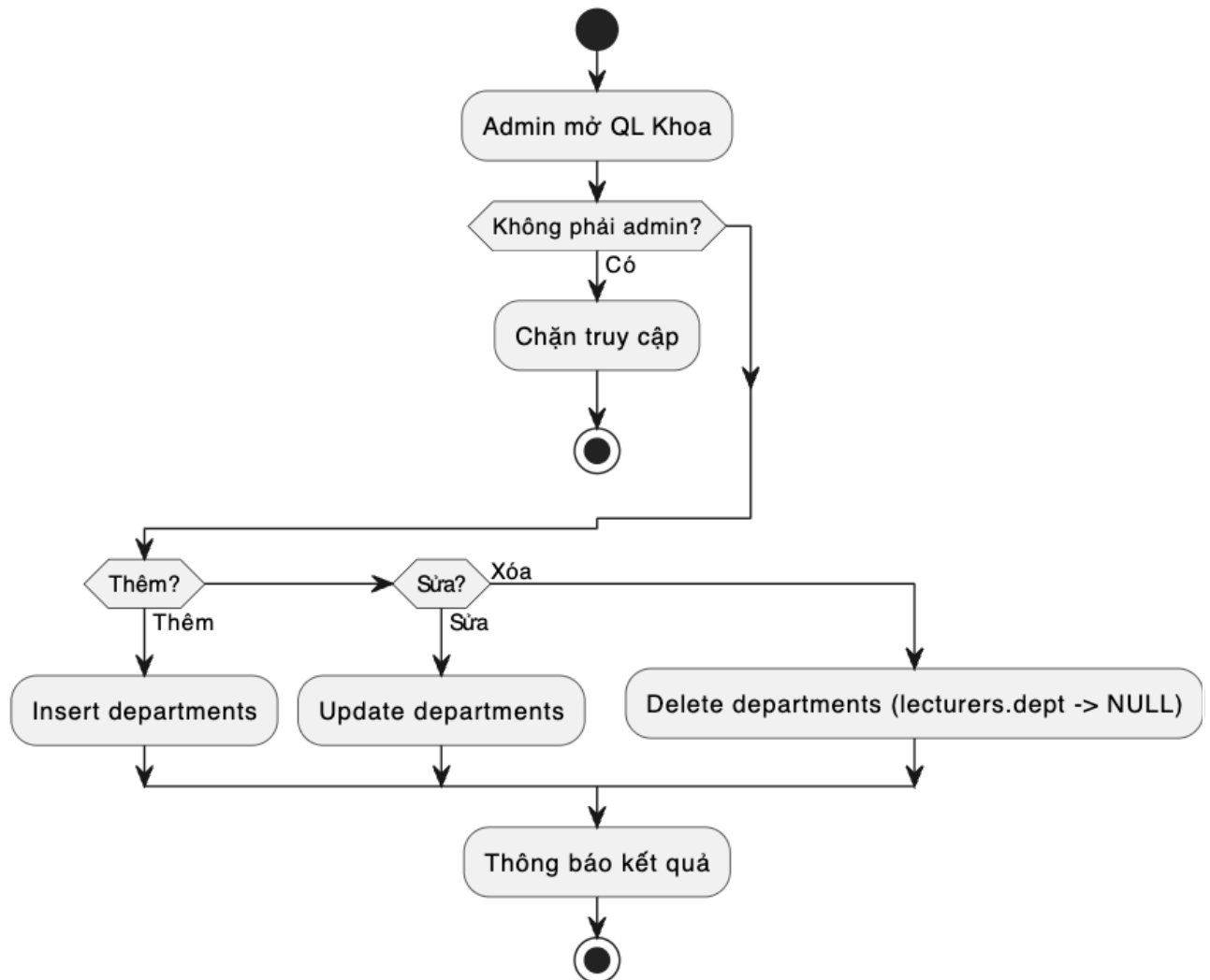
Hình 3-9: Biểu đồ hoạt động – Quản lý khoa/bộ môn (CRUD)
