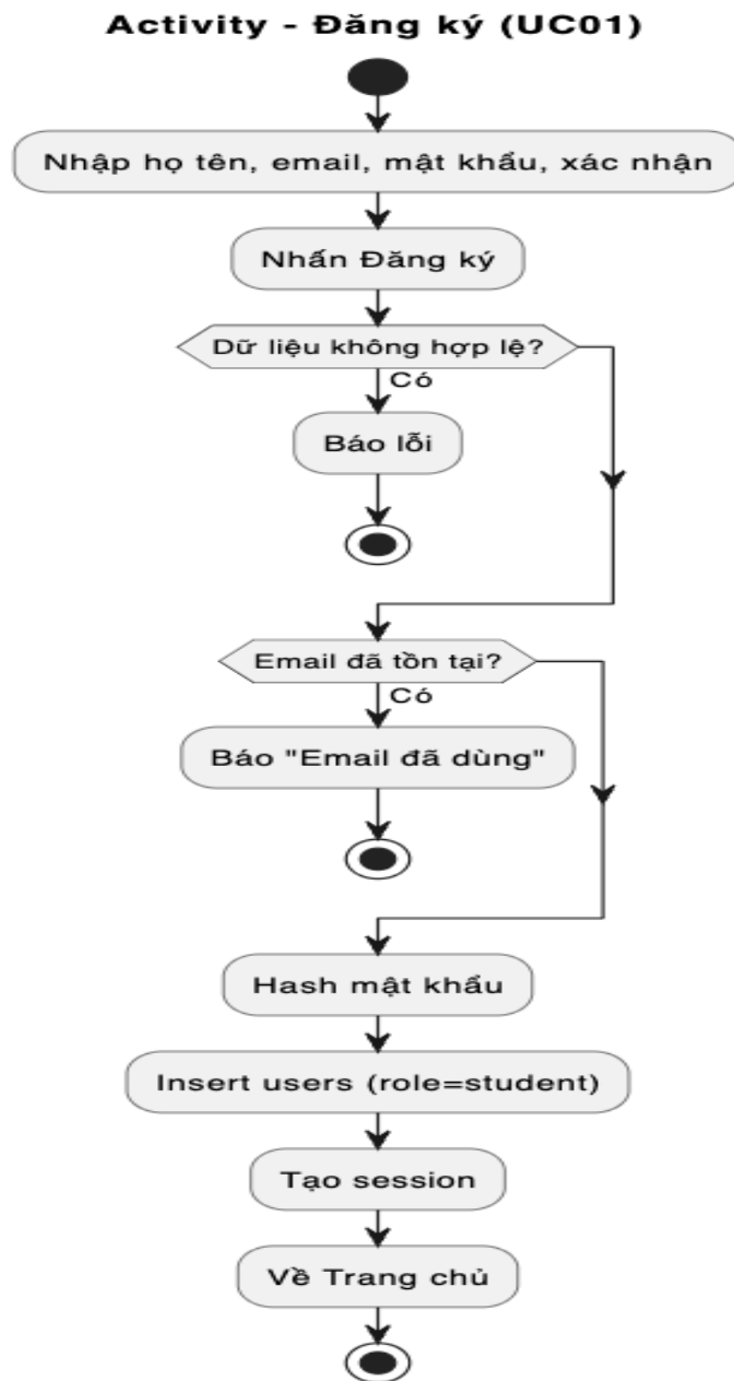
Hình 3-3: Biểu đồ hoạt động - Đăng ký tài khoản
