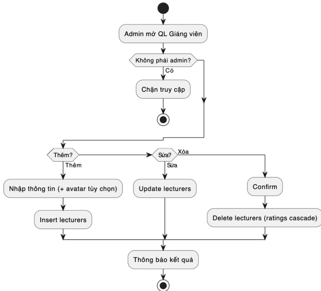
Hình 3-8: Biểu đồ hoạt động – Quản lý giảng viên (CRUD)
