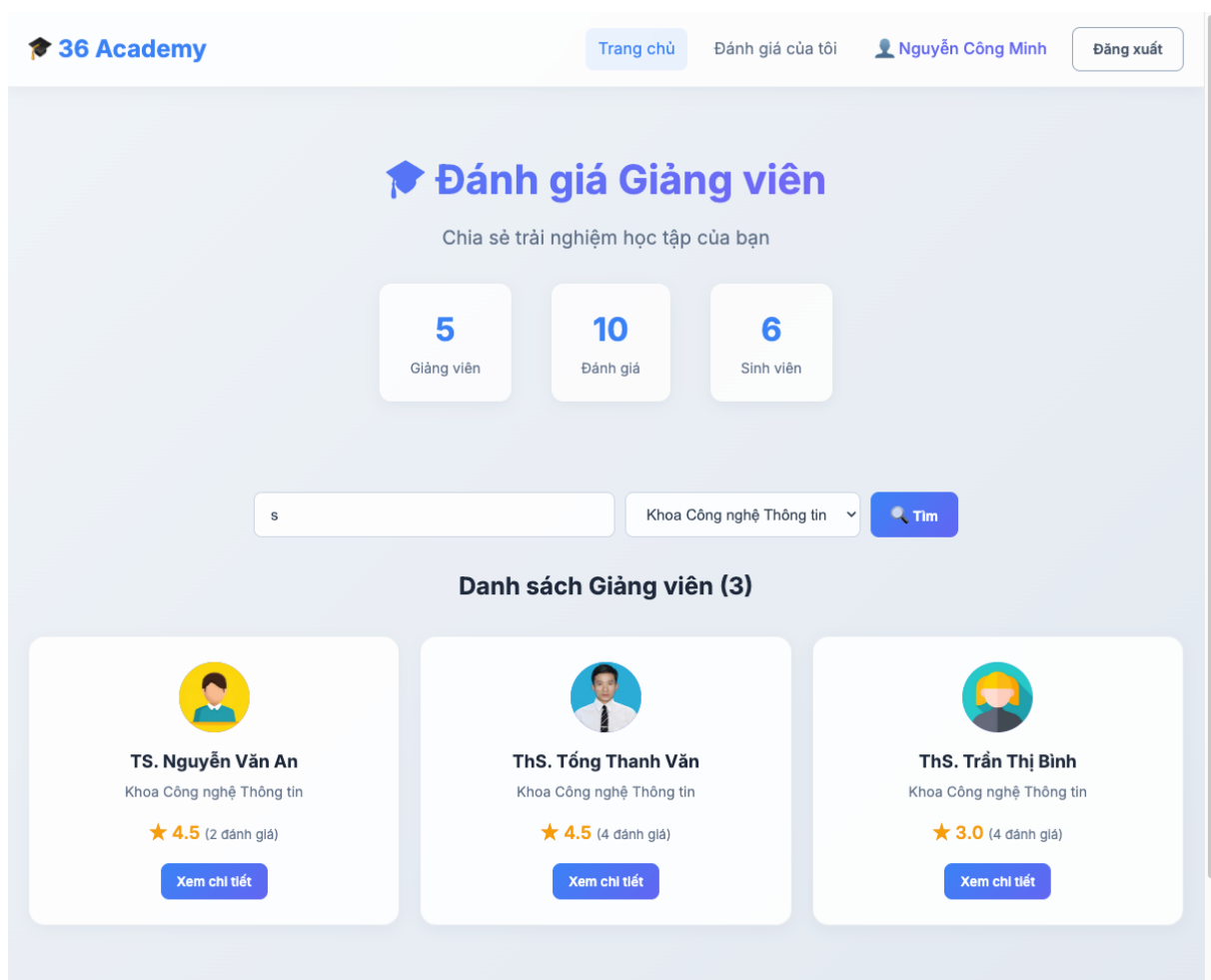
Hình 4-5: Kết quả tìm kiếm/lọc giảng viên theo từ khoá và theo khoa
