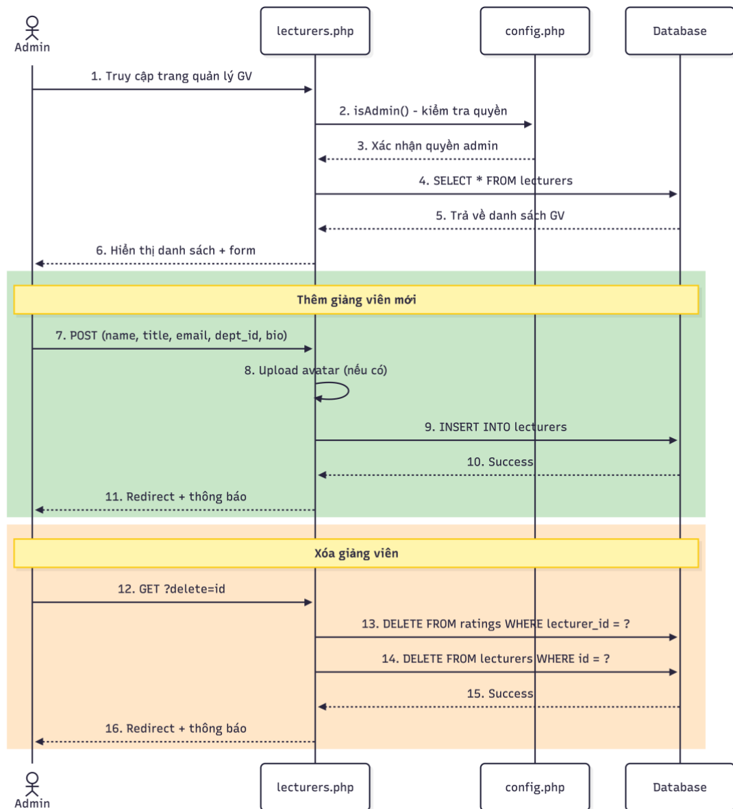
Hình 3-14: Biểu đồ tuần tự Quản lý giảng viên
