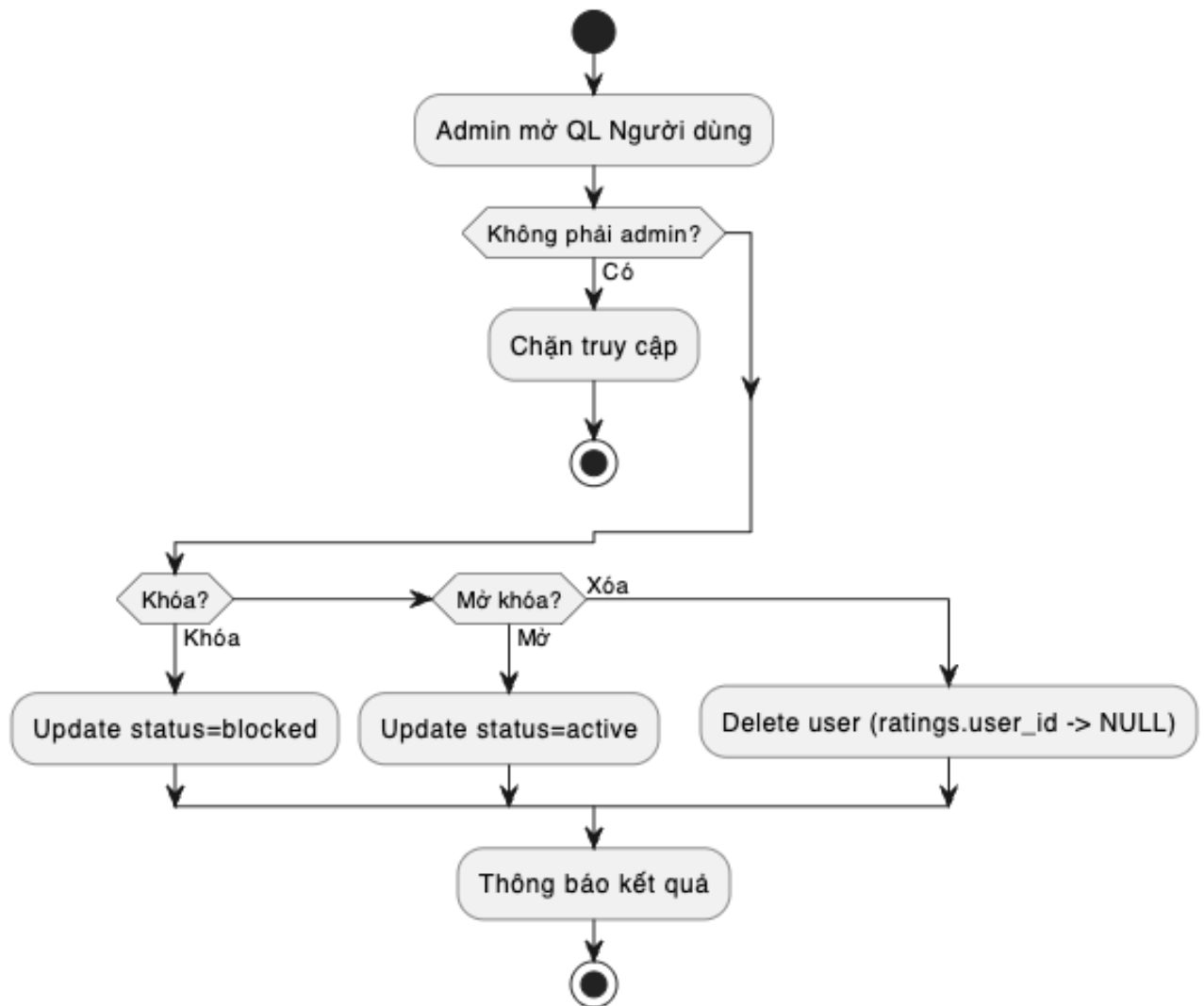
Hình 3-10: Biểu đồ hoạt động – Quản lý người dùng
