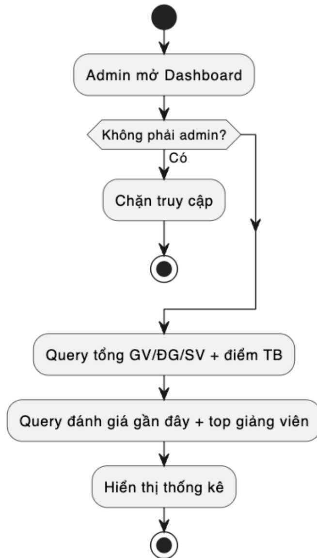
Hình 3-7: Biểu đồ hoạt động – Dashboard thống kê
