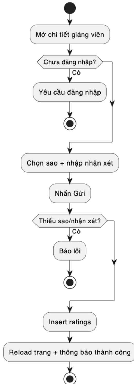
Hình 3-5: Biểu đồ hoạt động – Đánh giá giảng viên
