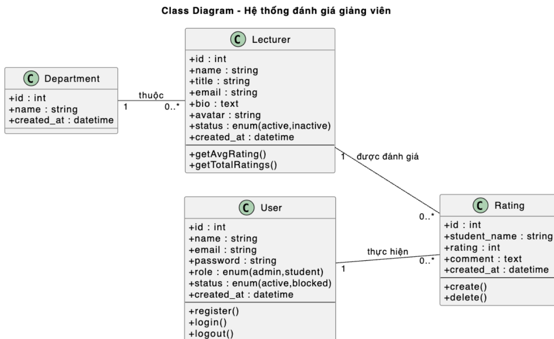
Hình 3-15: Biểu đồ lớp - Hệ thống đánh giá giảng viên
