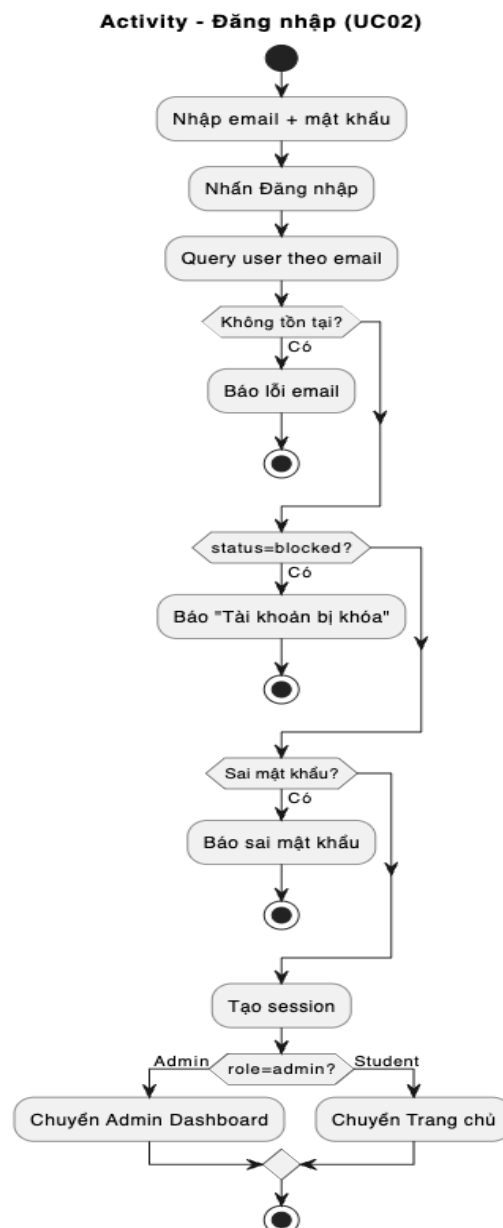
Hình 3-2: Biểu đồ hoạt động - Đăng nhập hệ thống
