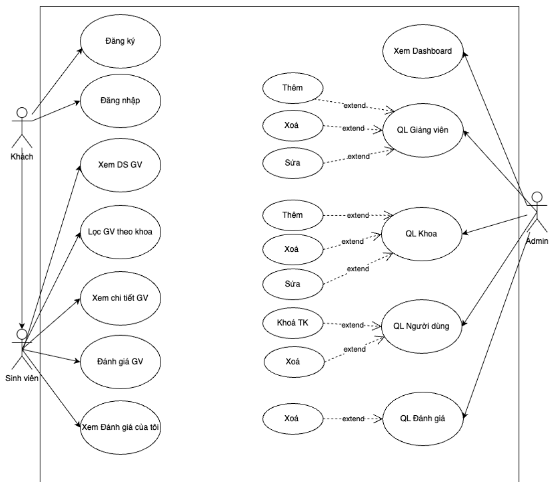
Hình 3-1: Use Case tổng quát của hệ thống
