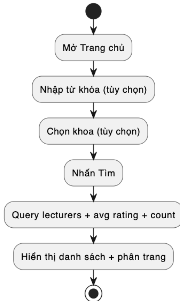
Hình 3-4: Biểu đồ hoạt động – Xem danh sách, tìm kiếm và lọc
