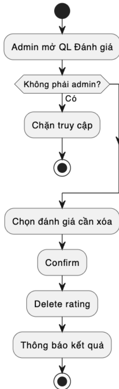
Hình 3-11: Biểu đồ hoạt động – Quản lý đánh giá
