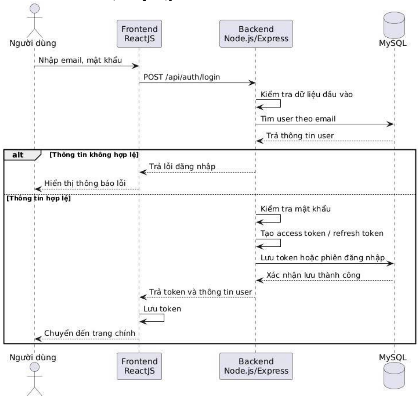
Hình 3-12: Biểu đồ tuần tự Đăng nhập
