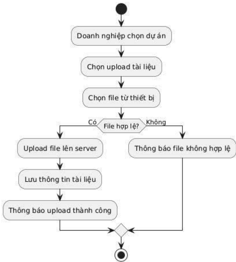
Hình 3-10: Biểu đồ hoạt động upload tài liệu dự án
