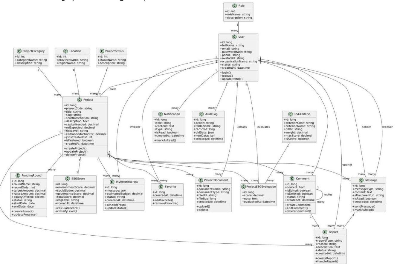
Hình 3-15: Biểu đồ lớp - Hệ thống Green Investment Intelligence Platform
