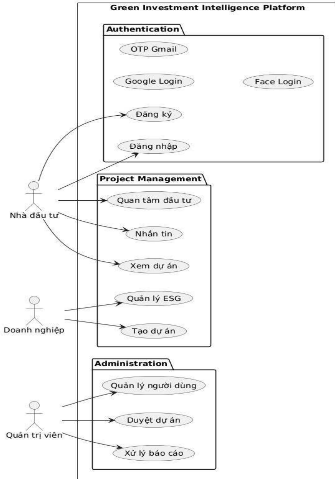
Hình 3-1: Use Case tổng quát của hệ thống
