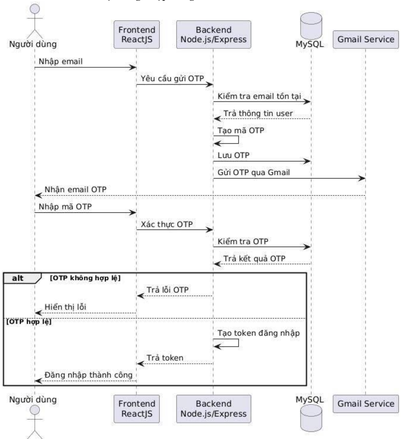
Hình 3-13: Biểu đồ tuần tự Đăng nhập bằng OTP Gmail
