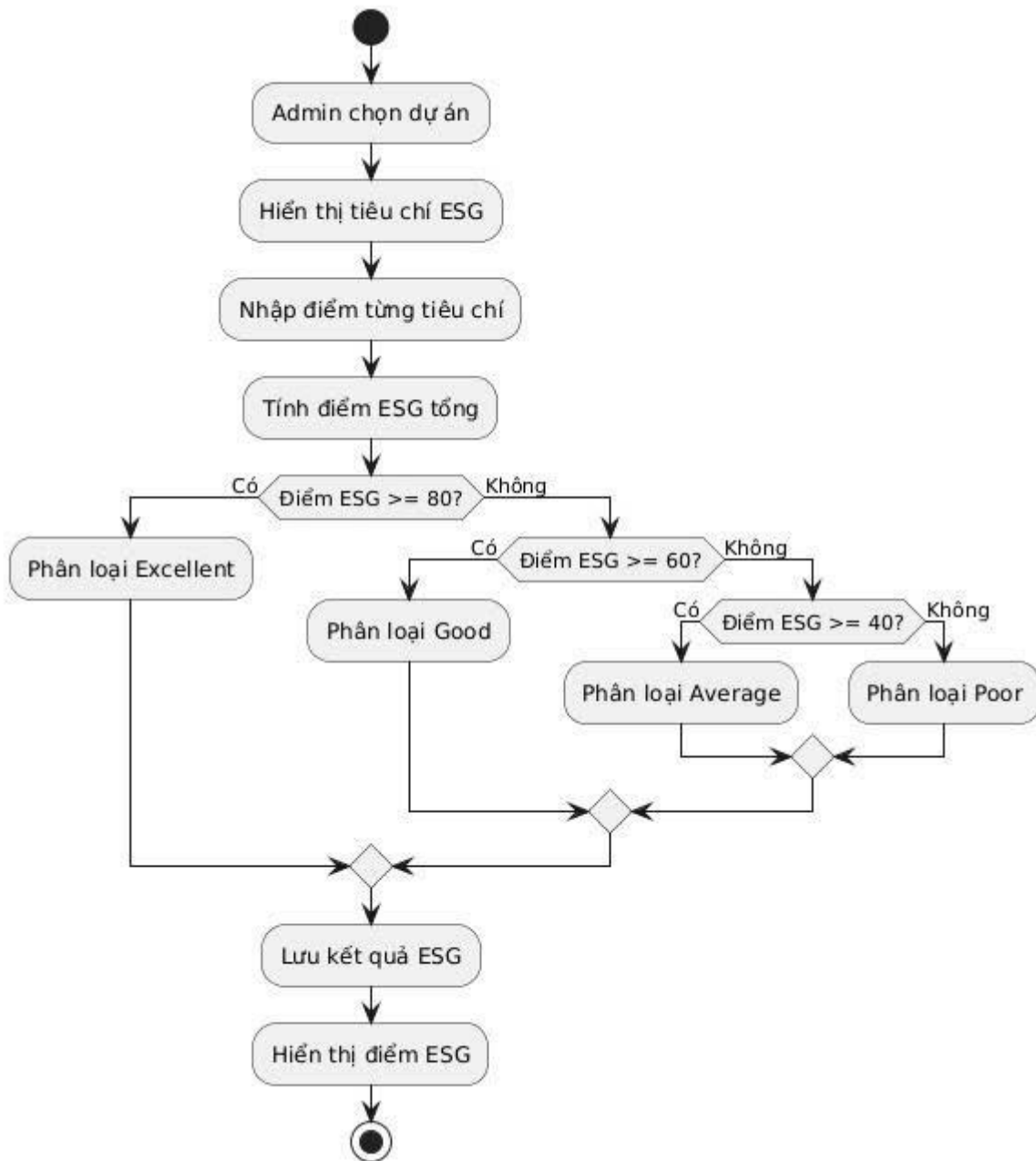
Hình 3-6: Biểu đồ hoạt động chấm điểm ESG
