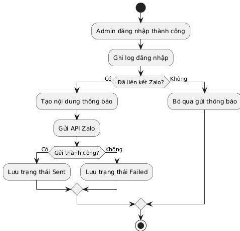
Hình 3-11: Biểu đồ hoạt động gửi thông báo Zalo
