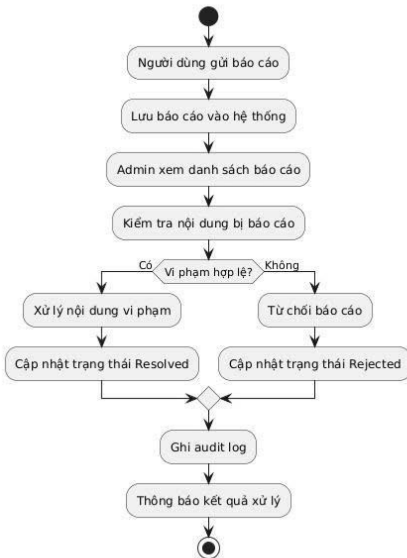
Hình 3-8: Biểu đồ hoạt động xử lý báo cáo vi phạm
