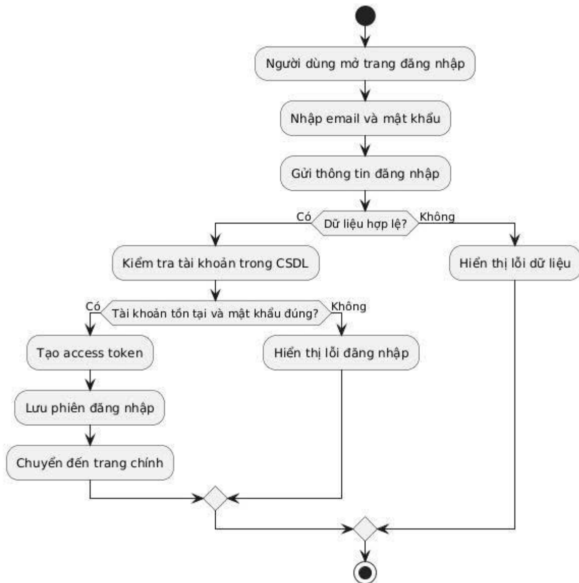
Hình 3-2: Biểu đồ hoạt động - Đăng nhập hệ thống
