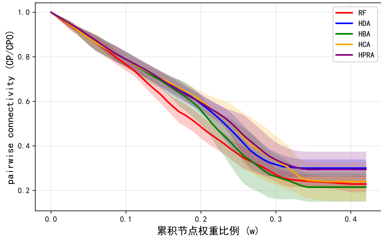
网络鲁棒性对比 - CP指标
