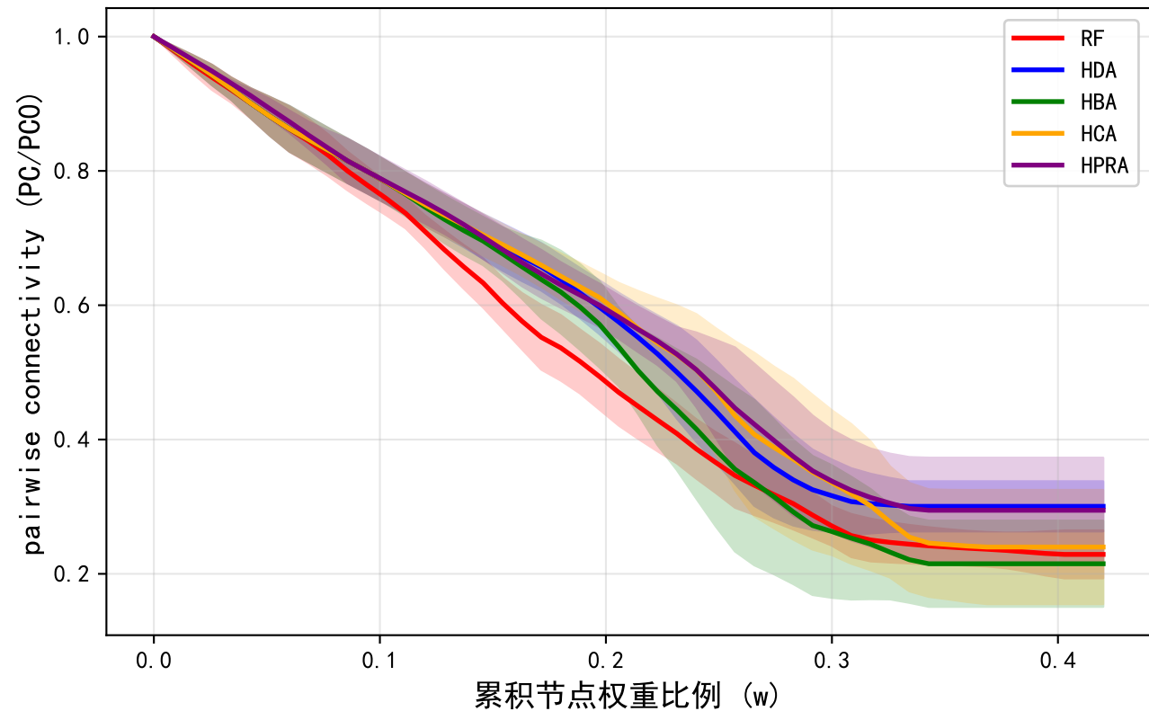
网络鲁棒性对比 - pc指标
