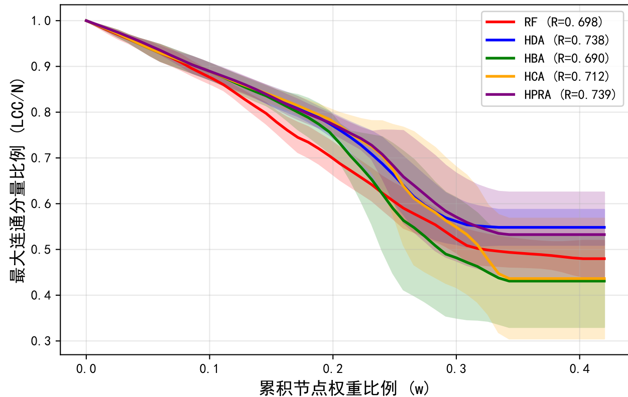
网络鲁棒性对比 - LCC指标
