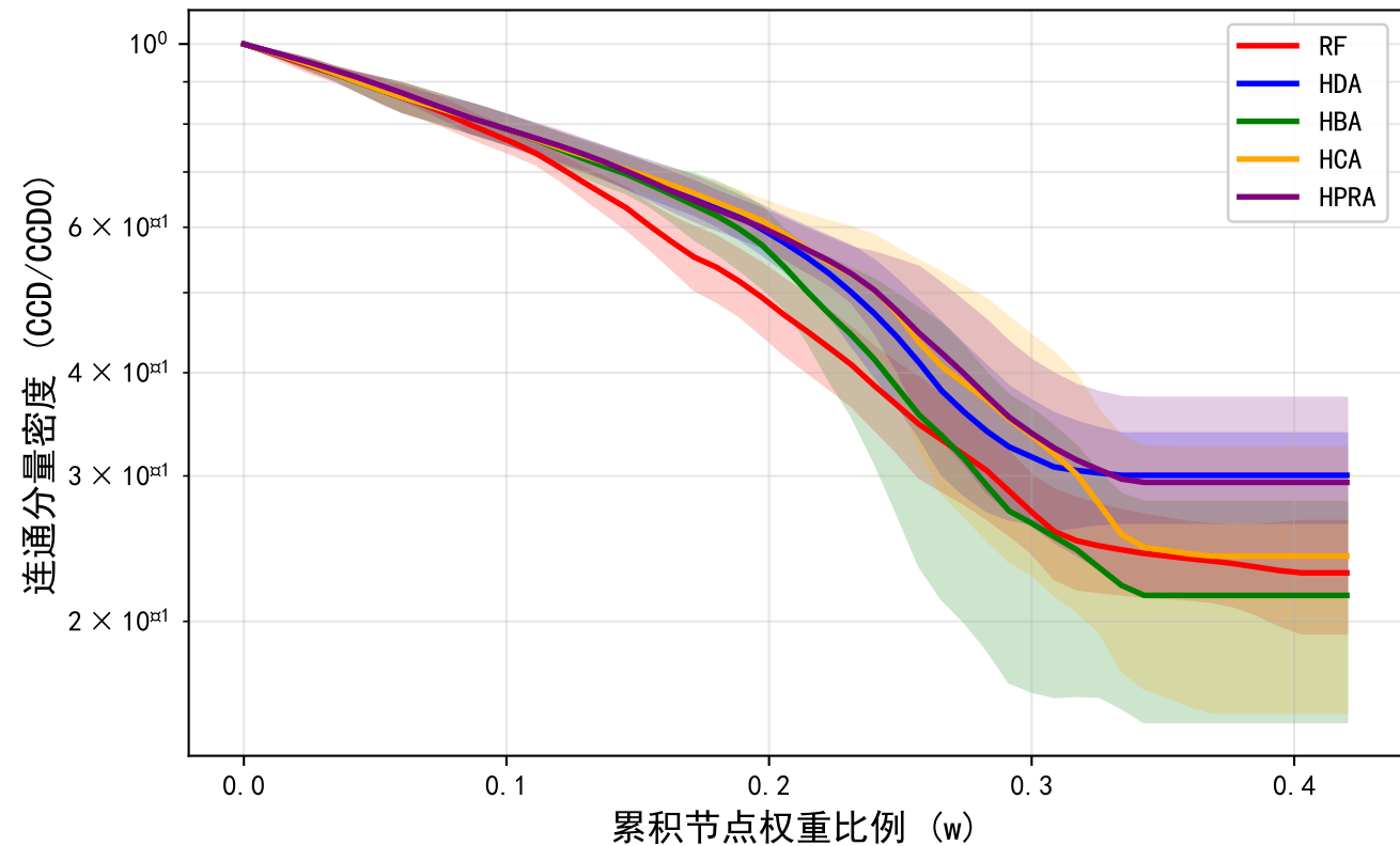
网络鲁棒性对比 - CCD指标
