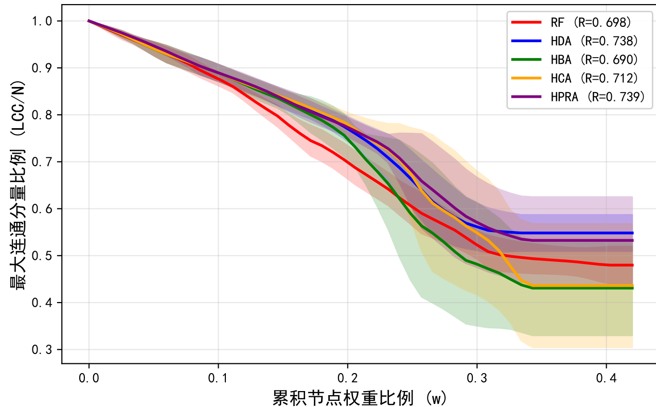
网络鲁棒性对比 - LCC指标
