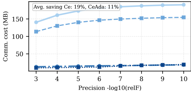
LogReg (real)
