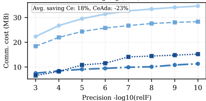
LogReg (real)
