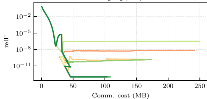
LogReg (real)
