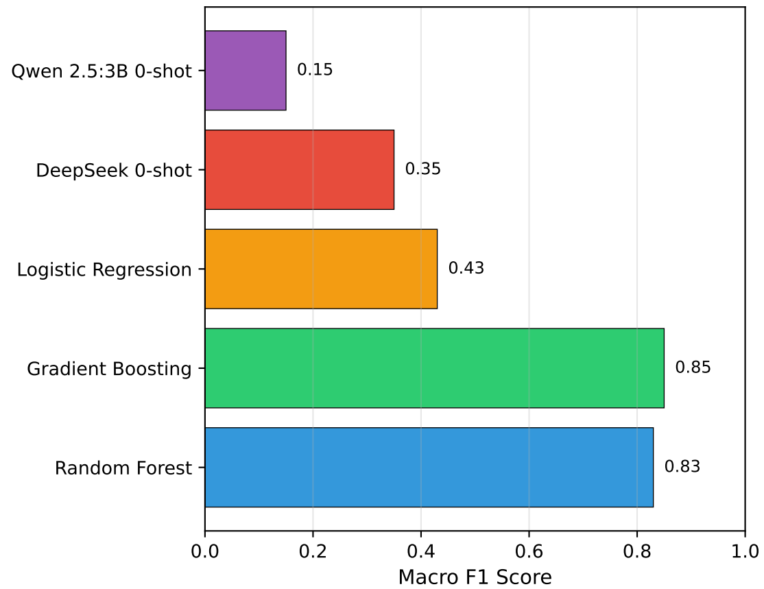
Macro F1 Score Comparison
