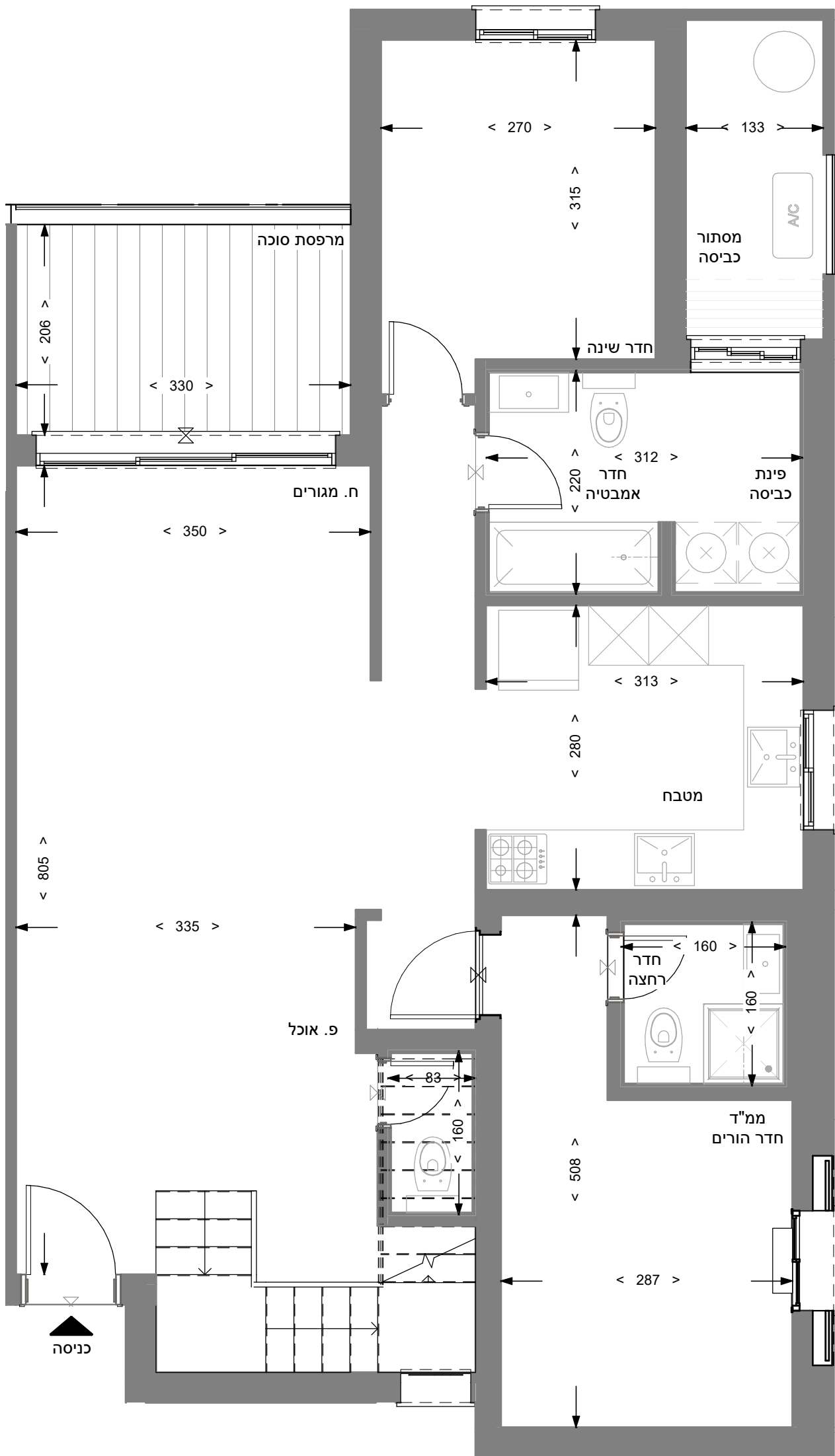
קומה 9
