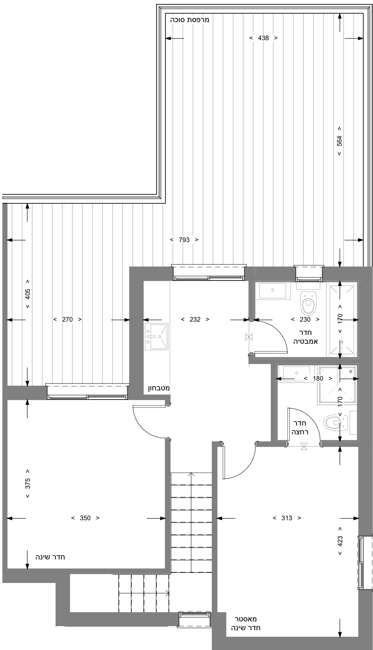
קומה 10
