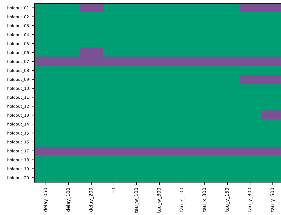
holdout TEB
