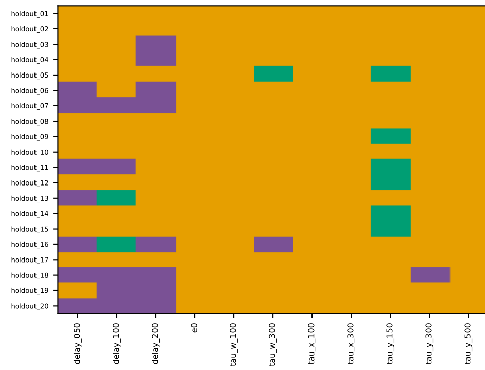
holdout DWA
