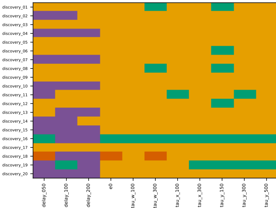
holdout DWA
