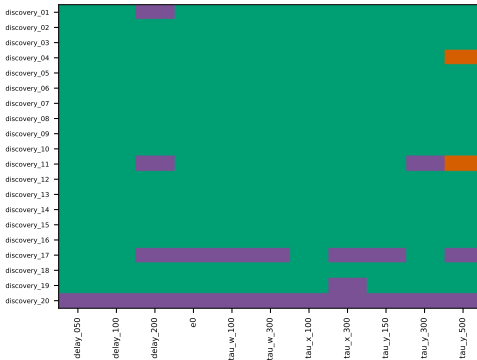
holdout TEB
