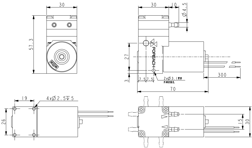
图 2 DPL30-24(12)BB 外形尺寸图
