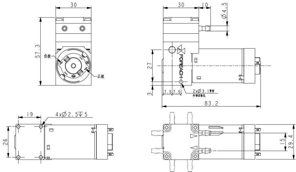
图 1 DPL30-24(12)DB 外形尺寸图
