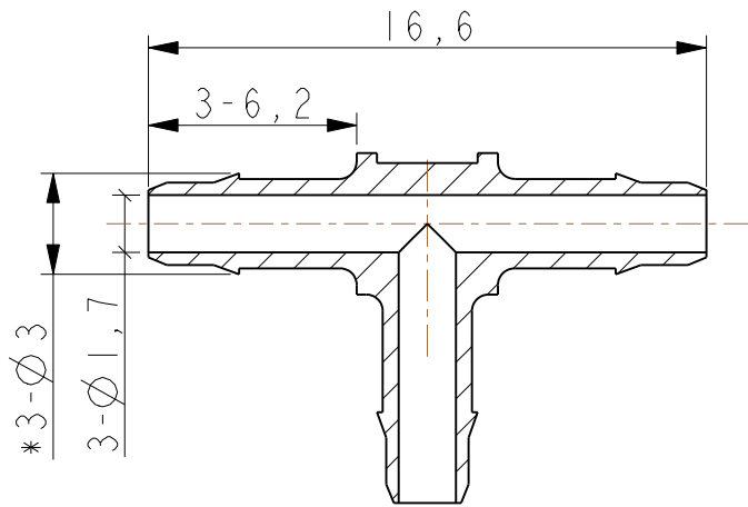
截面 A-A 比例 4,000
