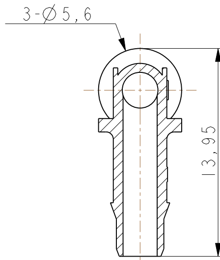
截面 B-B
