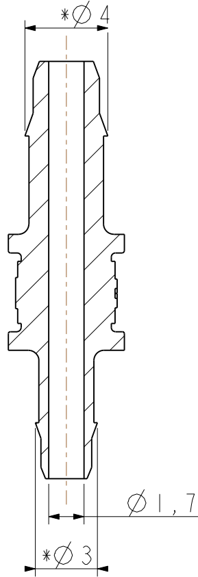
截面 A - A
