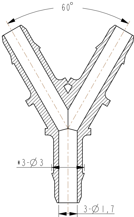
截面 A-A 比例 5,000
