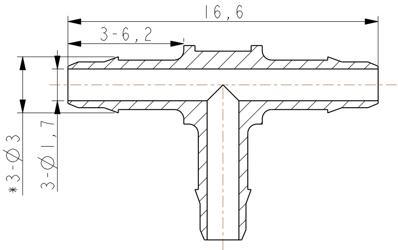
截面 A-A 比例 5,000
