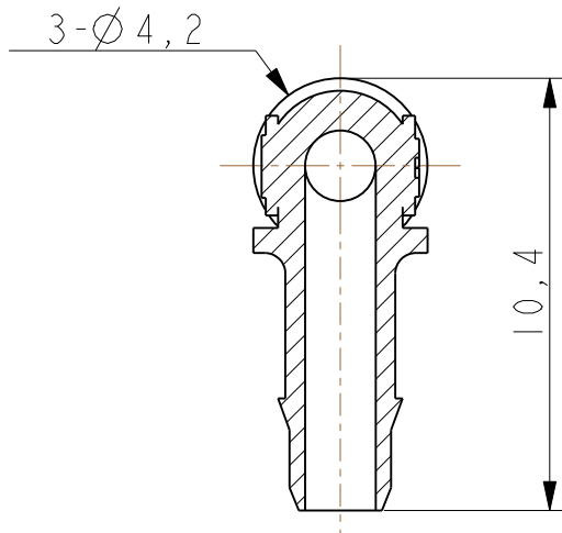
截面 B-B
