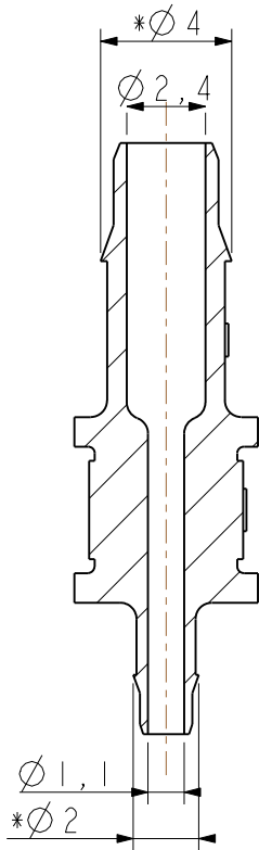
截面 A - A
