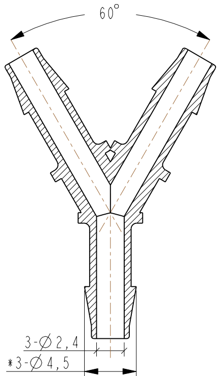
截面 A-A 比例 3,000
