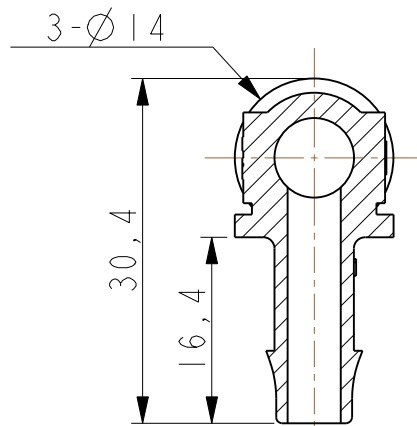
截面 B-B
