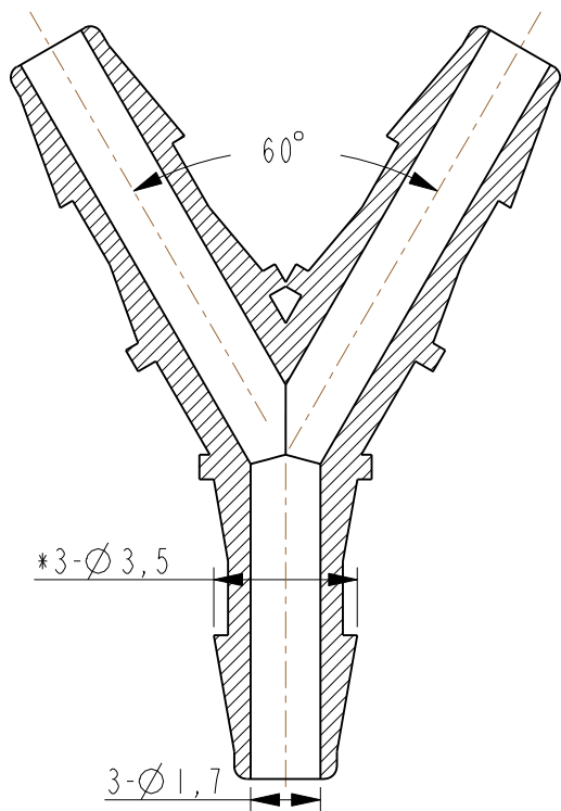
截面 A-A 比例 5,000
