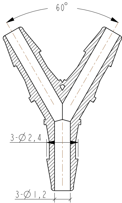
截面 A-A 比例 6,000
