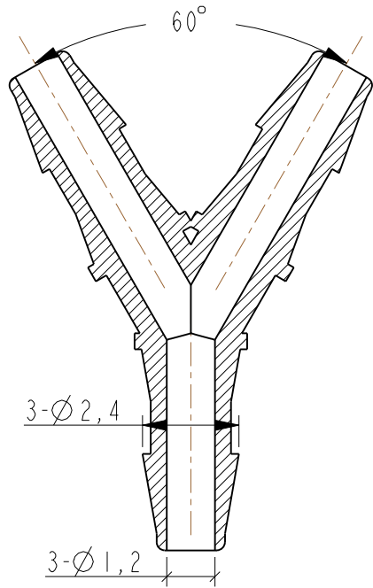
截面 A-A 比例 6,000
