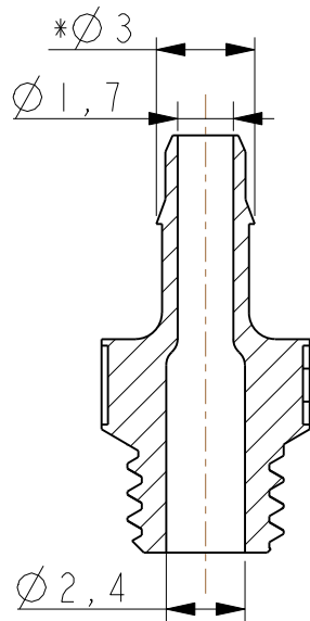
截面 B-B
