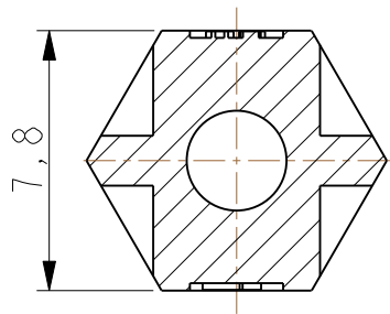
截面 B-B
