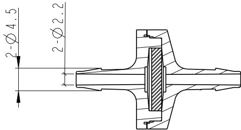
截面: B-B
