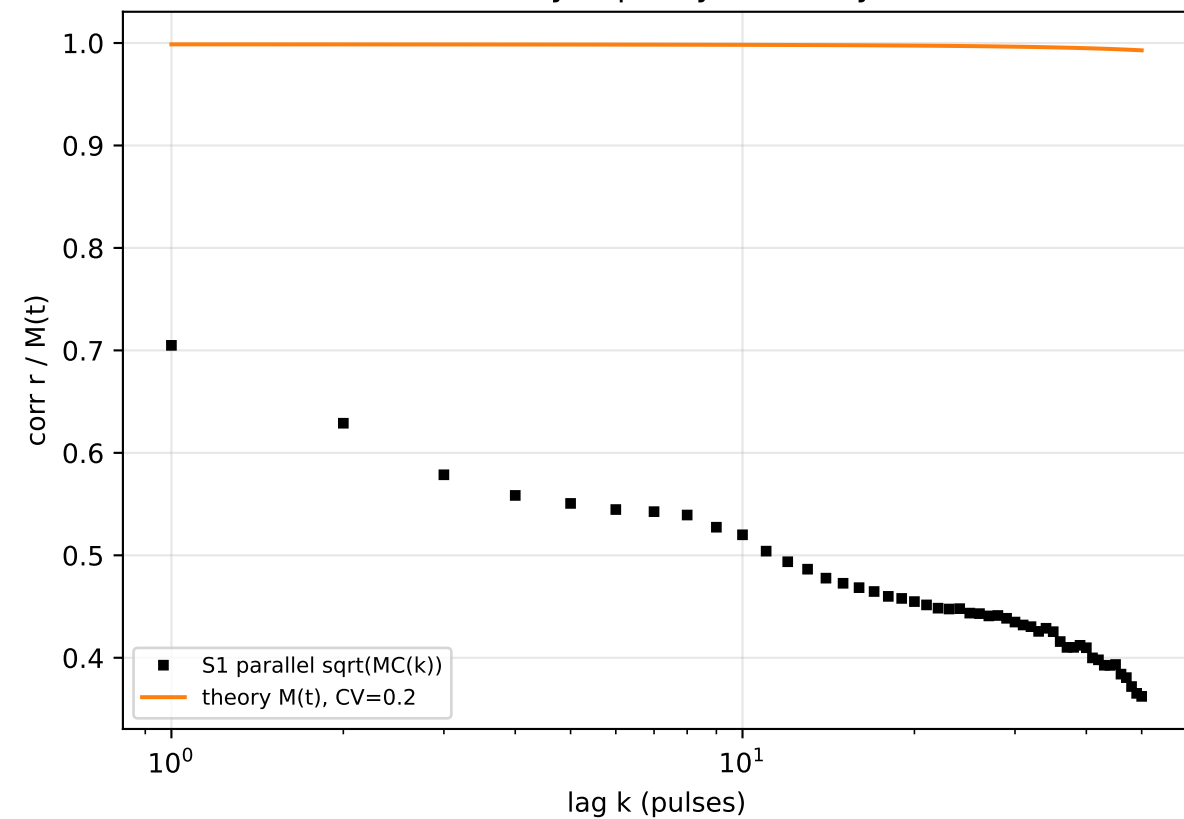
(d) S1 memory capacity vs theory kernel
