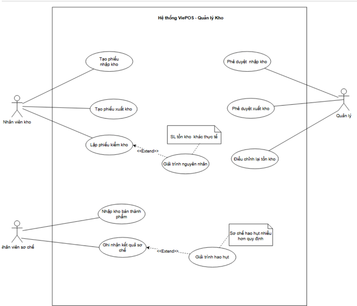
Hình 5-1. Usecase quản lý kho
