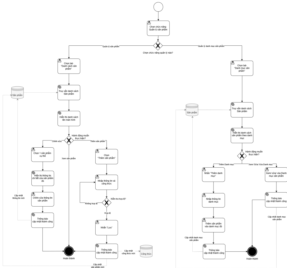
Hình. BPMN Quản lý sản phẩm
