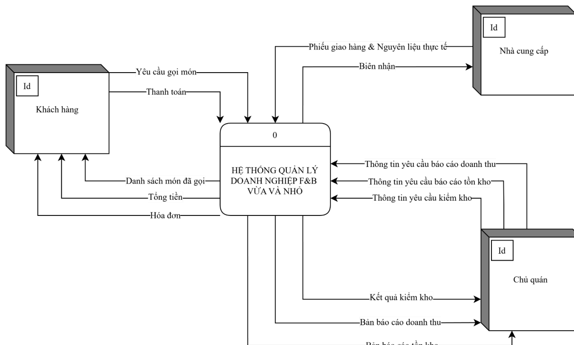
Hình 2-2. Sơ đồ DFD context
