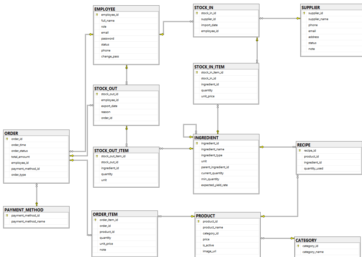
Hình 4-1. Sơ đồ quan hệ thực thể
