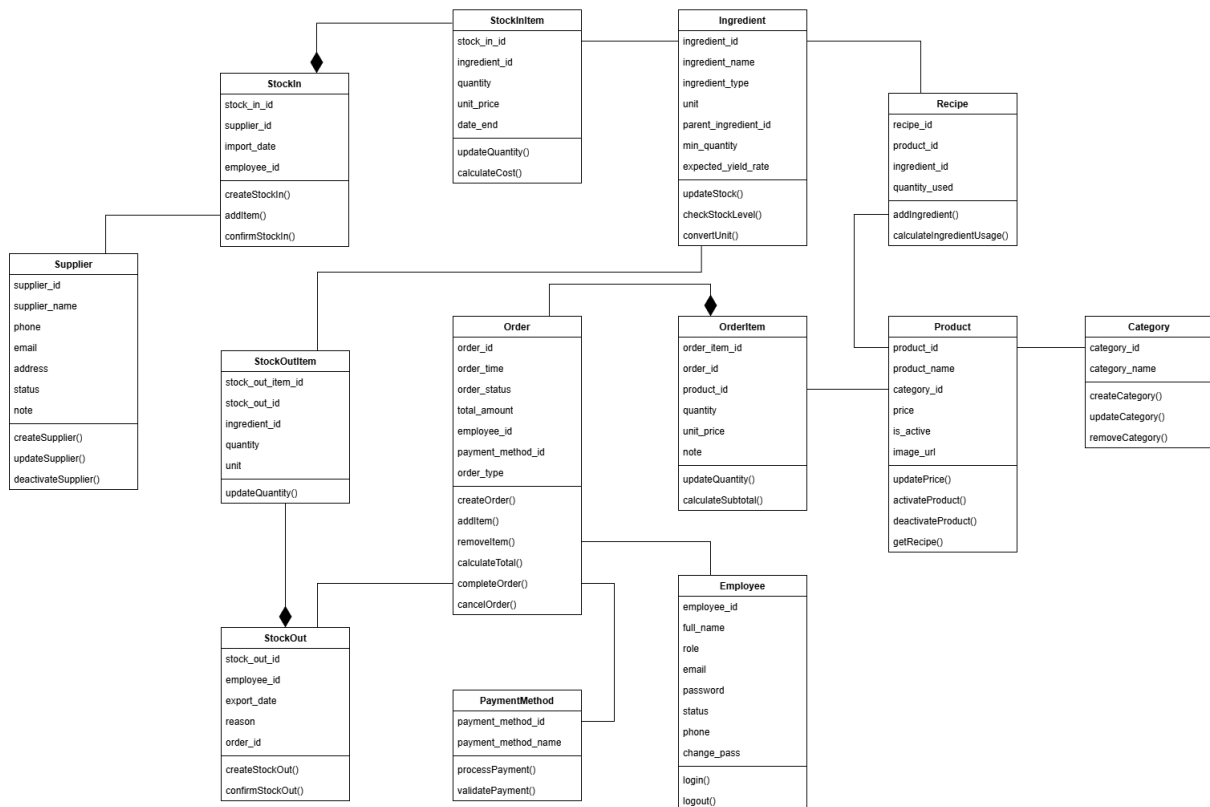
Hình 5-2. Class Diagram của hệ thống quản lý bán hàng và kho nguyên liệu quán cà phê
