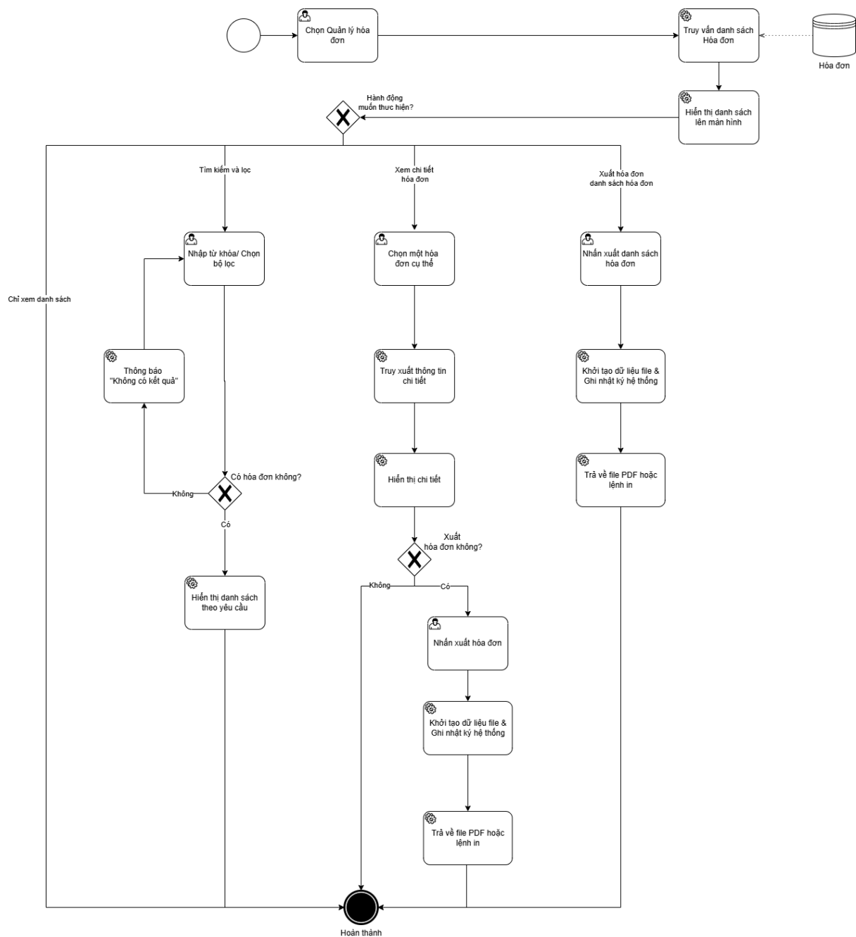
Hình. BPMN Quản lý hóa đơn
