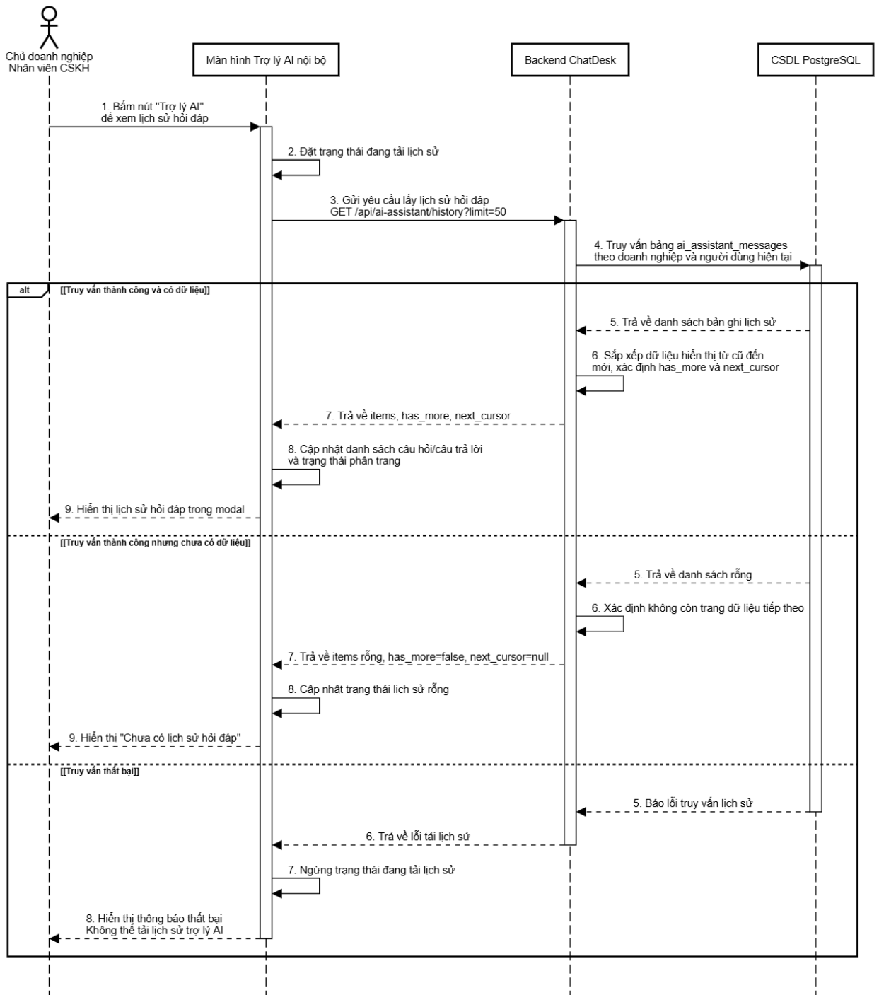
Hình 2.32: Biểu đồ tuần tự Xem lịch sử hỏi đáp
