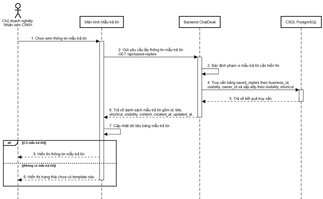
Hình 2.28: Biểu đồ tuần tự Xem thông tin mẫu trả lời
