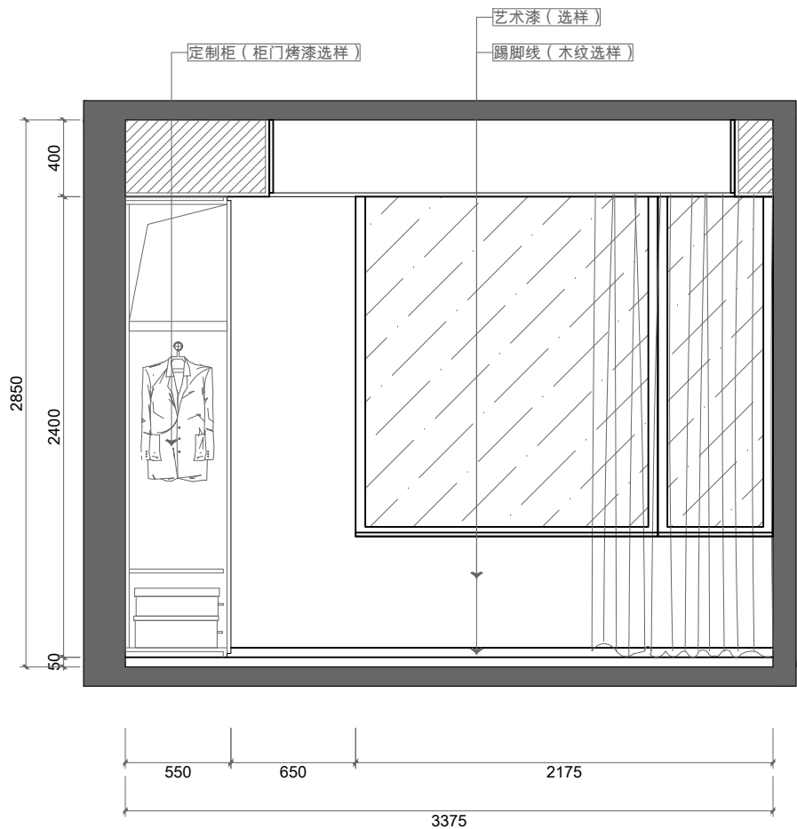
主臥C立面图 1:35
