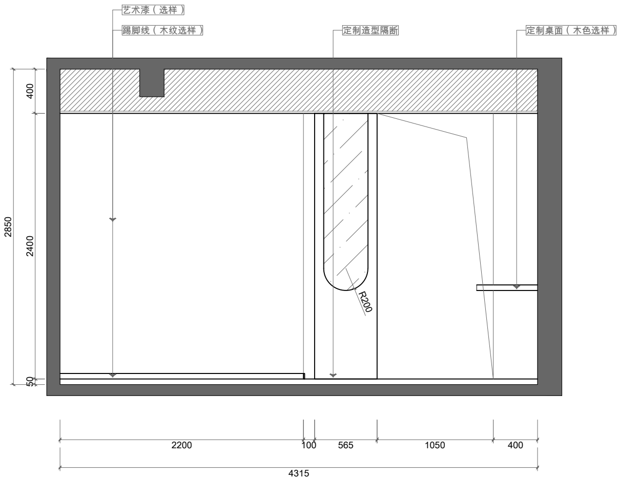
主卧室A立面图 1:35
