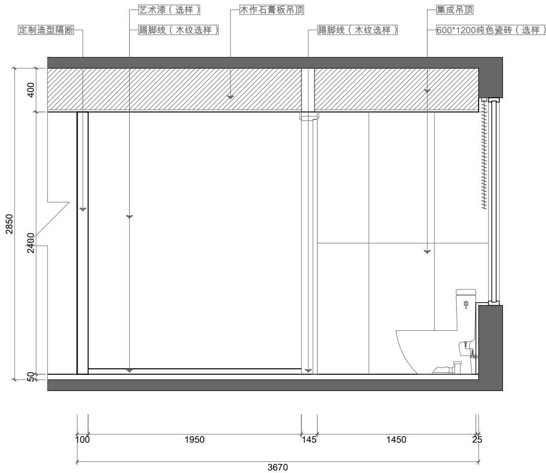
主卧室干区、主卫D立面图 1:35
