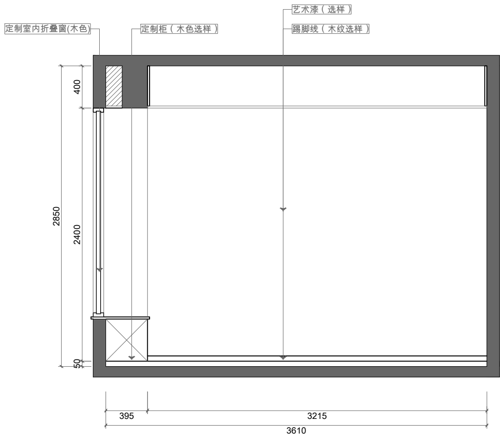
书房D立面图 1:35
