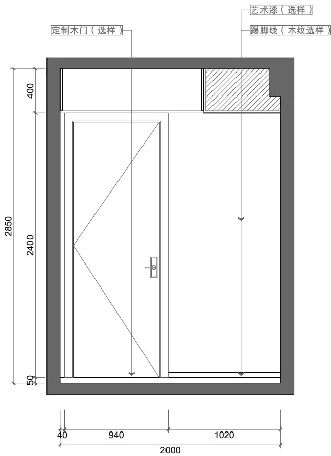
书房A立面图 1:35
