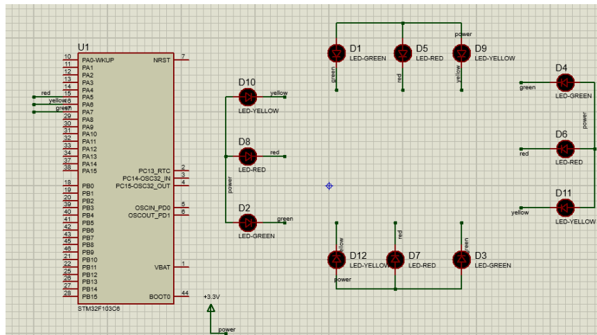
Hình 5: Proteus Schematic for Exercise 3.
