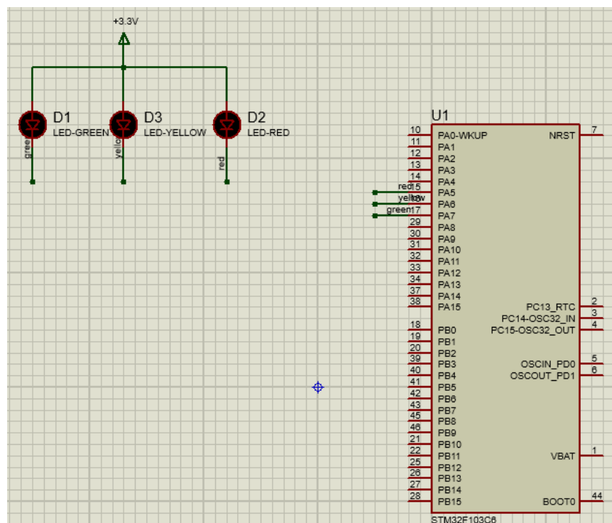
Hình 3: Proteus Schematic for Exercise 2.
