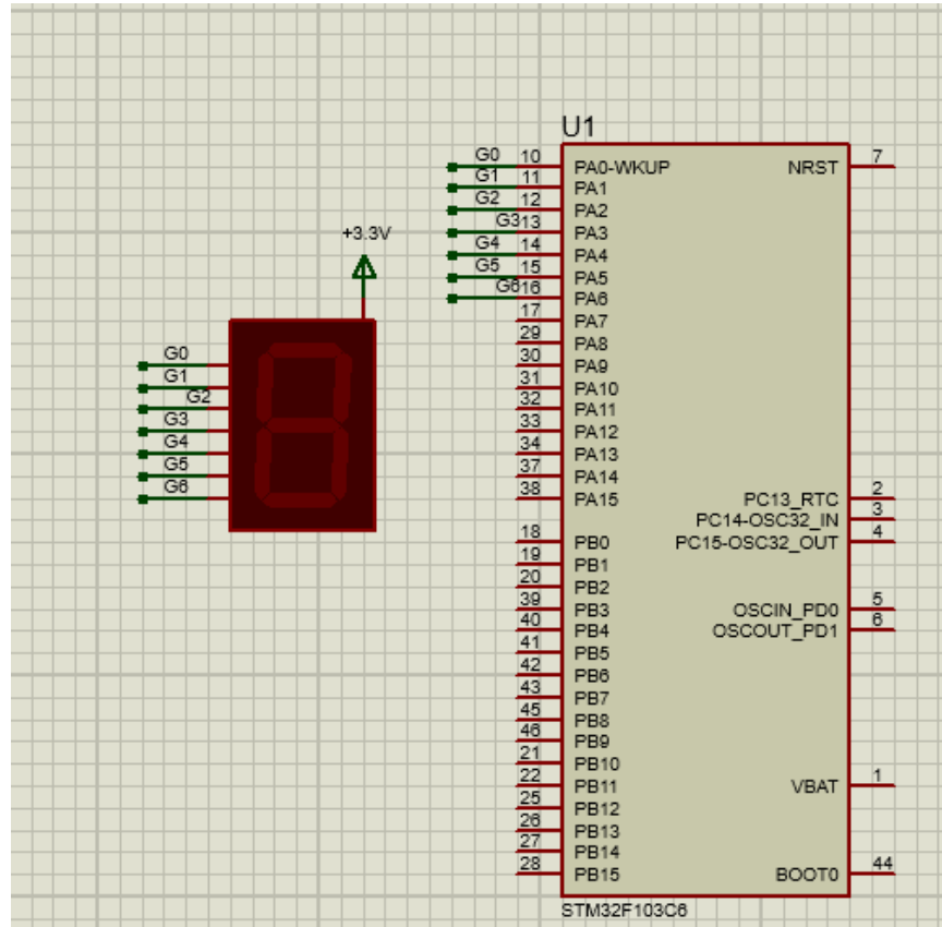
Hình 7: Proteus Schematic for Exercise 4.
