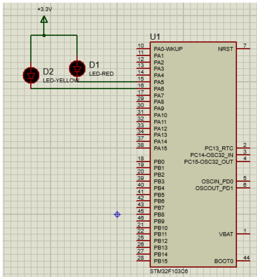
Hình 2: Proteus Schematic for Exercise 1.
