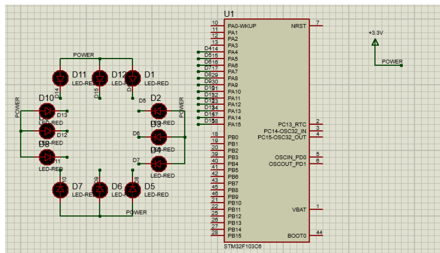
Hình 9: Proteus Schematic for Exercise 6.
