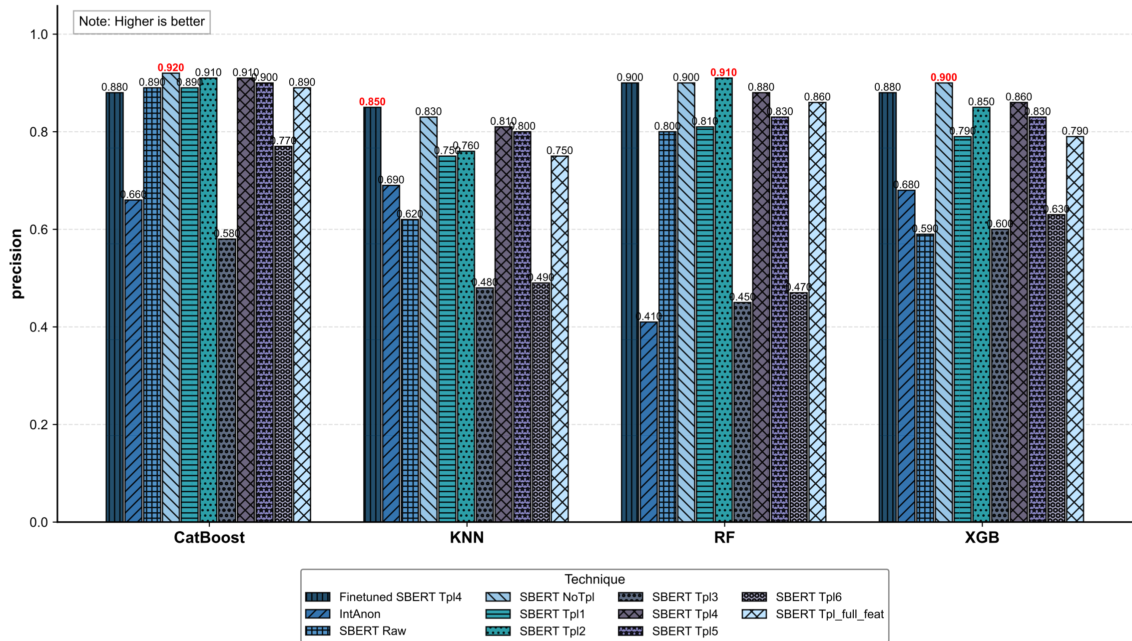
Task: ec | Metric: precision
