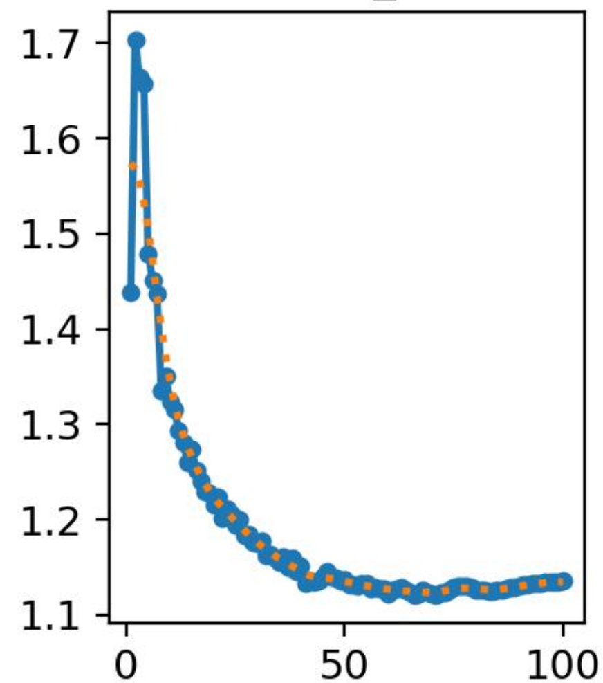
val/box_loss
