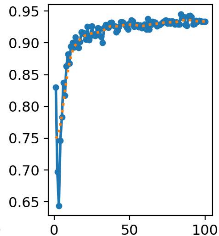
metrics/precision(B)
