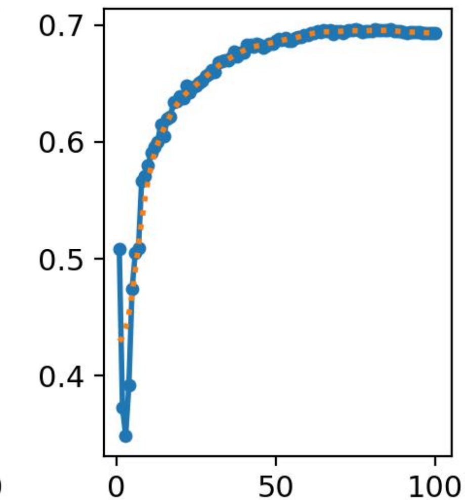
metrics/mAP50-95(B)
